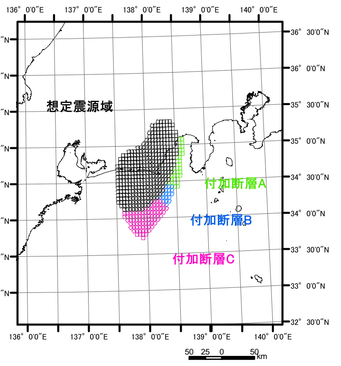
想定震源域と付加断層の位置
