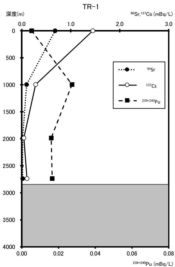
図 2-2 各調査点における海水中の各核種の鉛直分布図 (2/2)
