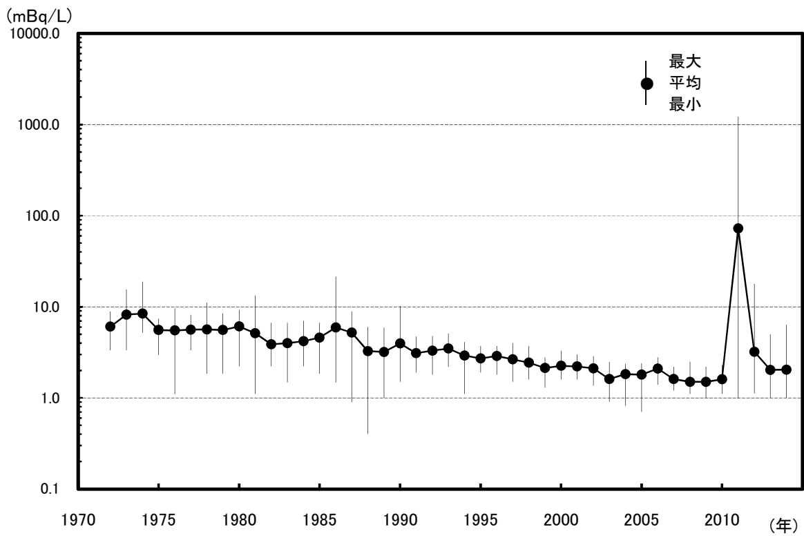
図 1-6 日本近海海水中の ^{137}\text{Cs} の経年変化
