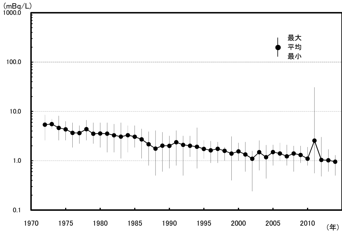
図 1-5 日本近海海水中の ^{90}\text{Sr} の経年変化
