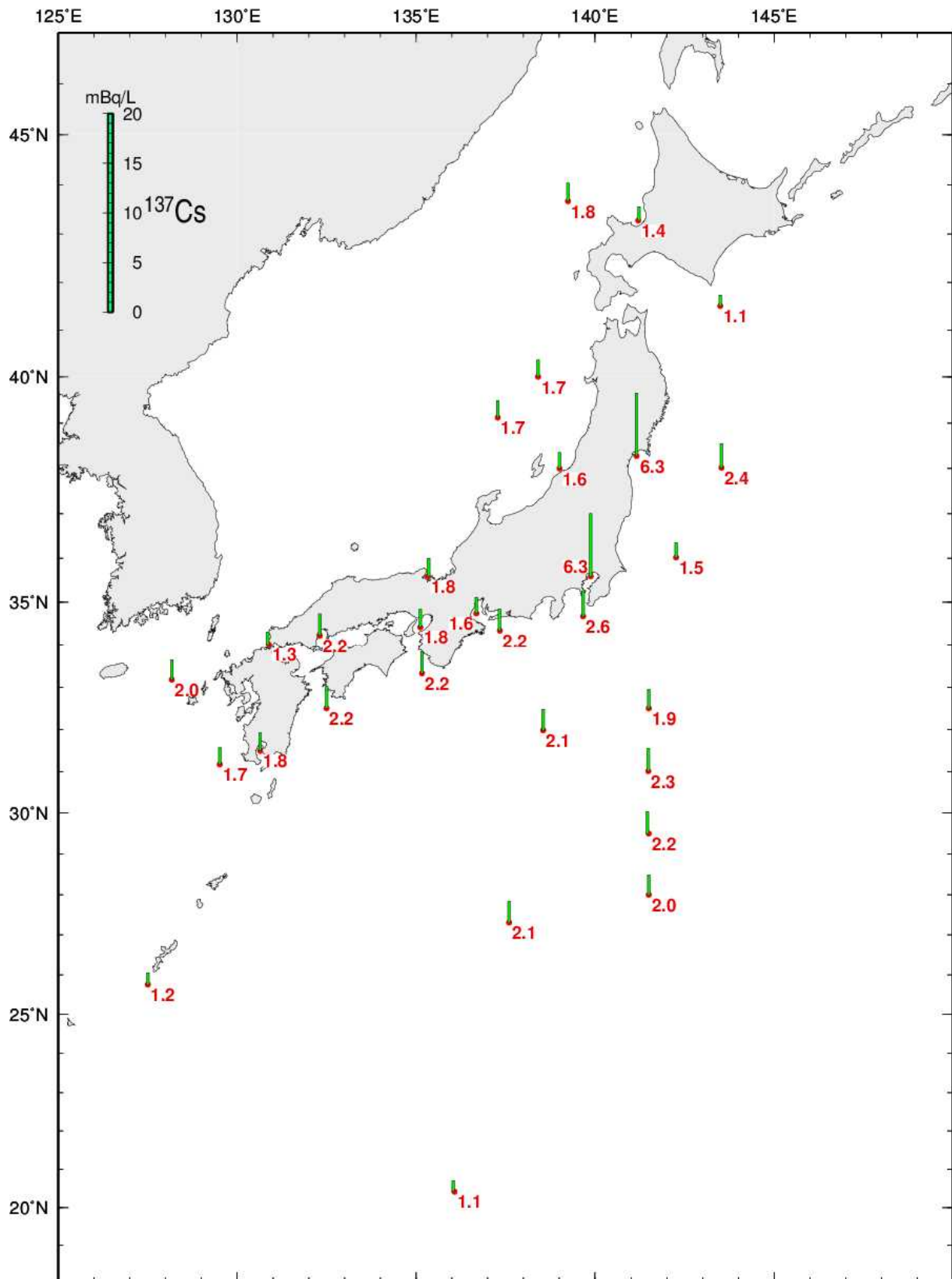
図 1-3 平成 26 年日本近海放射能調査結果－海水中の ^{137}\text{Cs}
