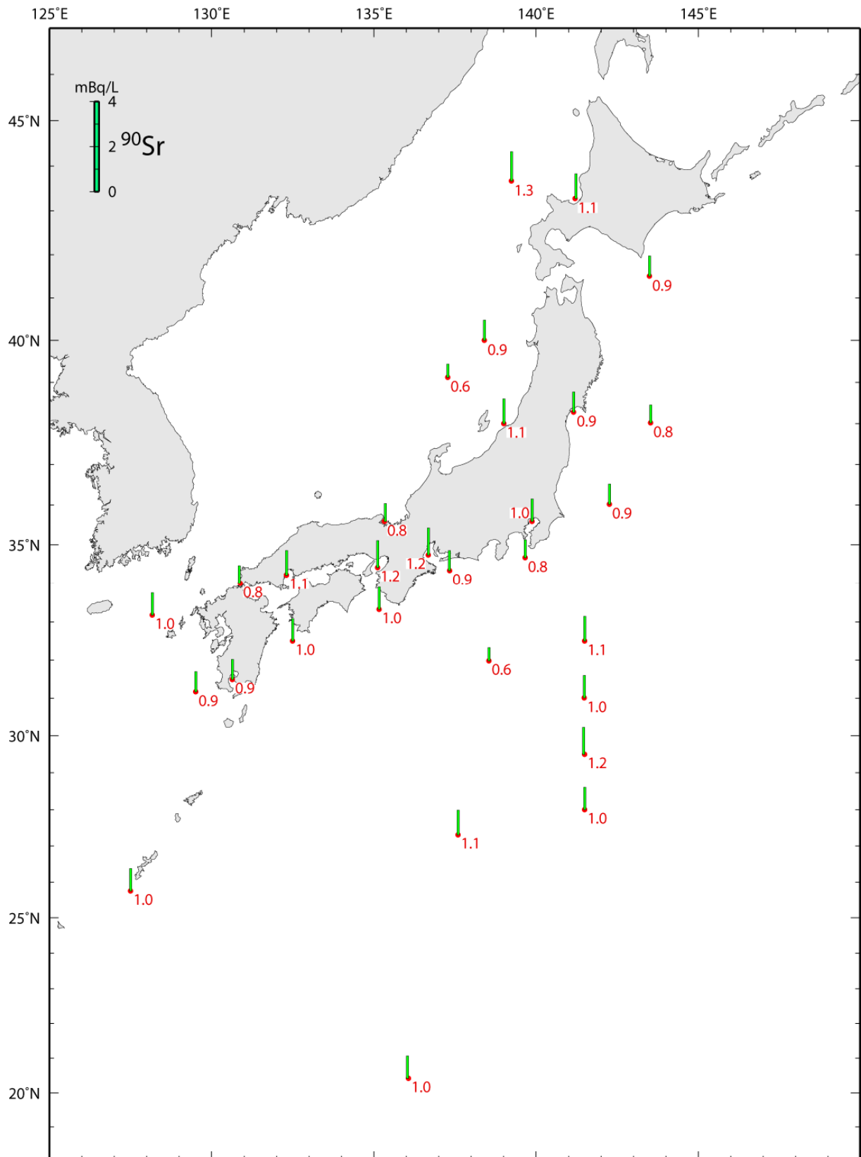
図 1-2 平成 26 年日本近海放射能調査結果—海水中の ^{90}\text{Sr}
