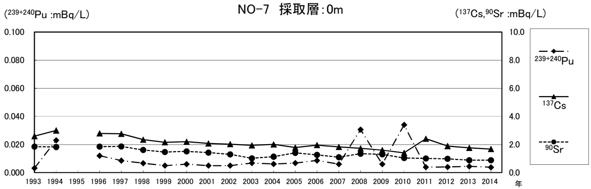
図 2-3 各調査点における海水中の各核種の経年変化図 (2/5)
