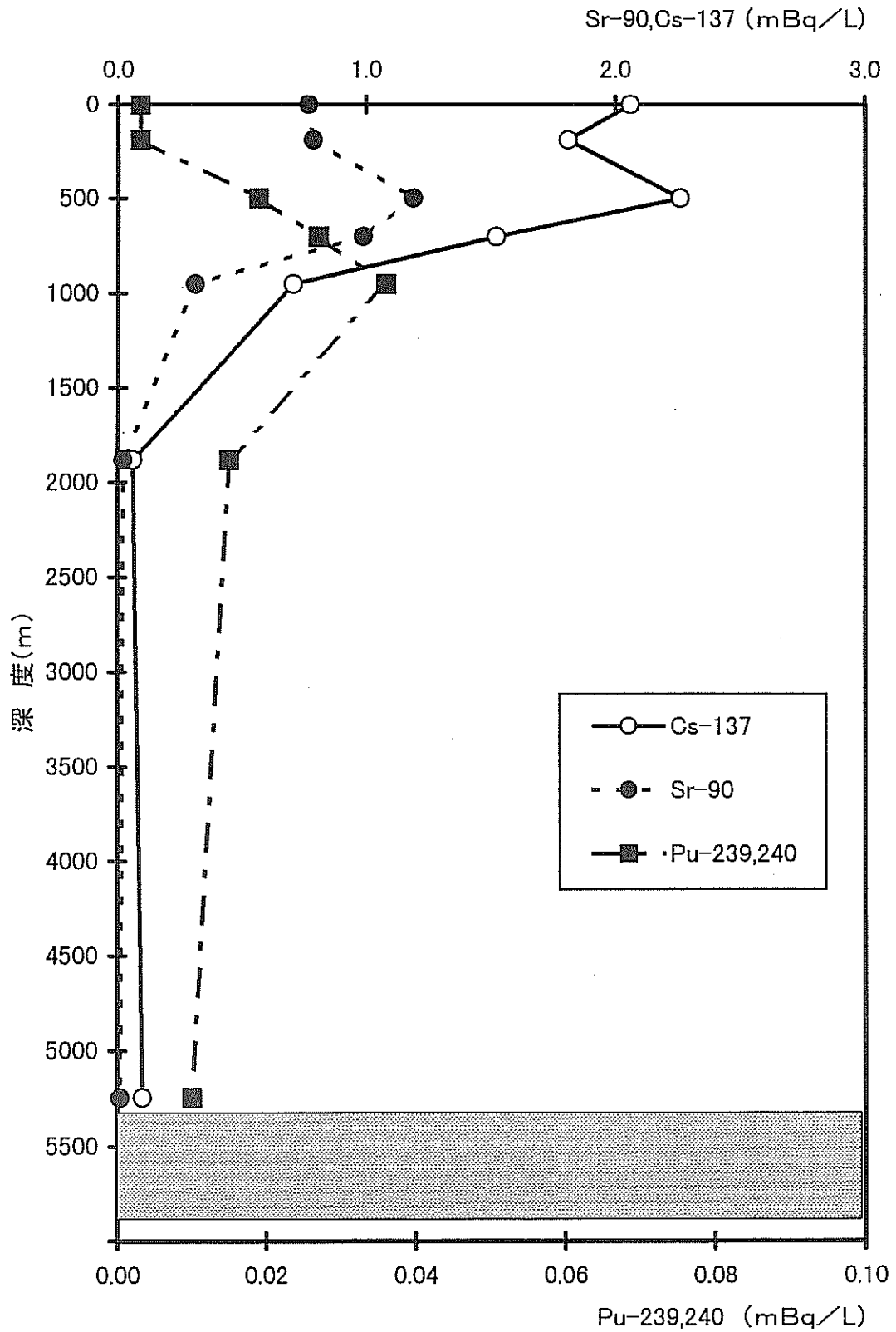
図3-2 測点Aにおける海水中的の各核種の鉛直分布
