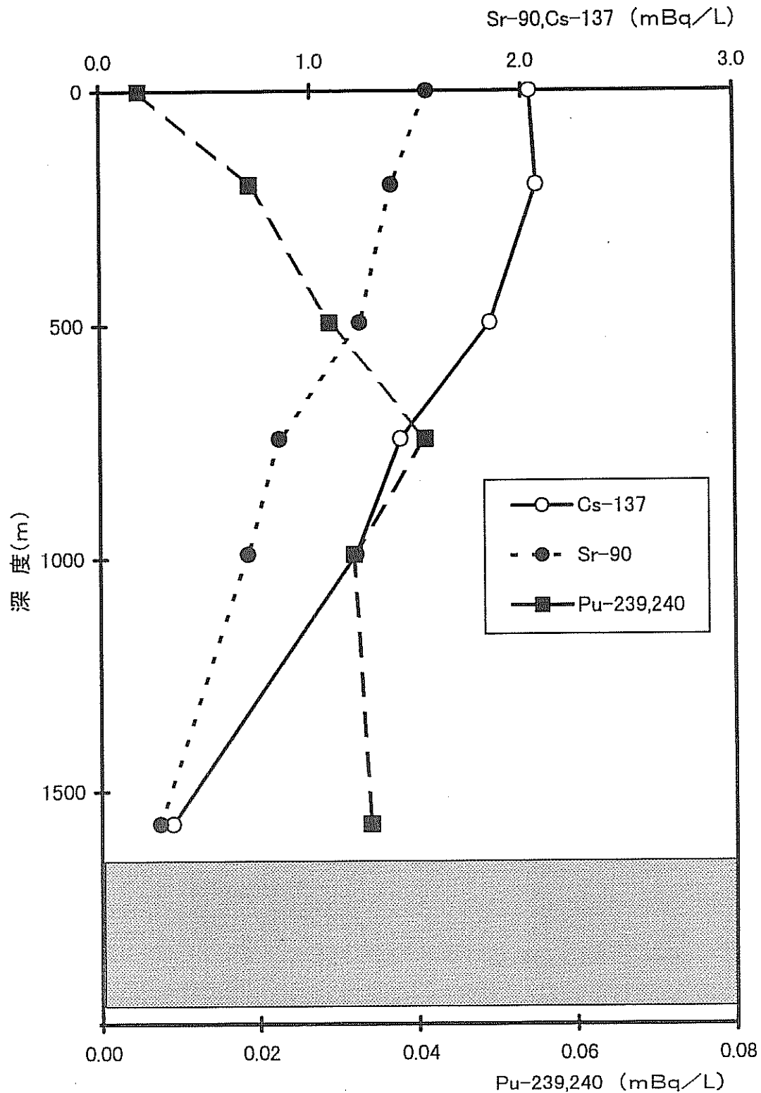
図3-5 測点NO-2における海水中的各核種の鉛直分布
