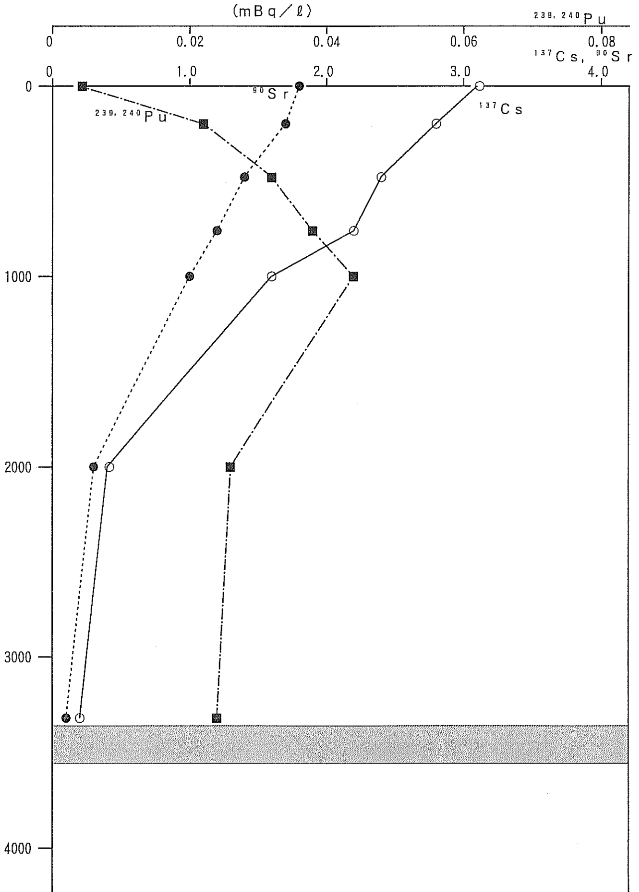
図3-9 測点NO-6における海水中のPu-239,240、Cs-137及びSr-90の鉛直分布
