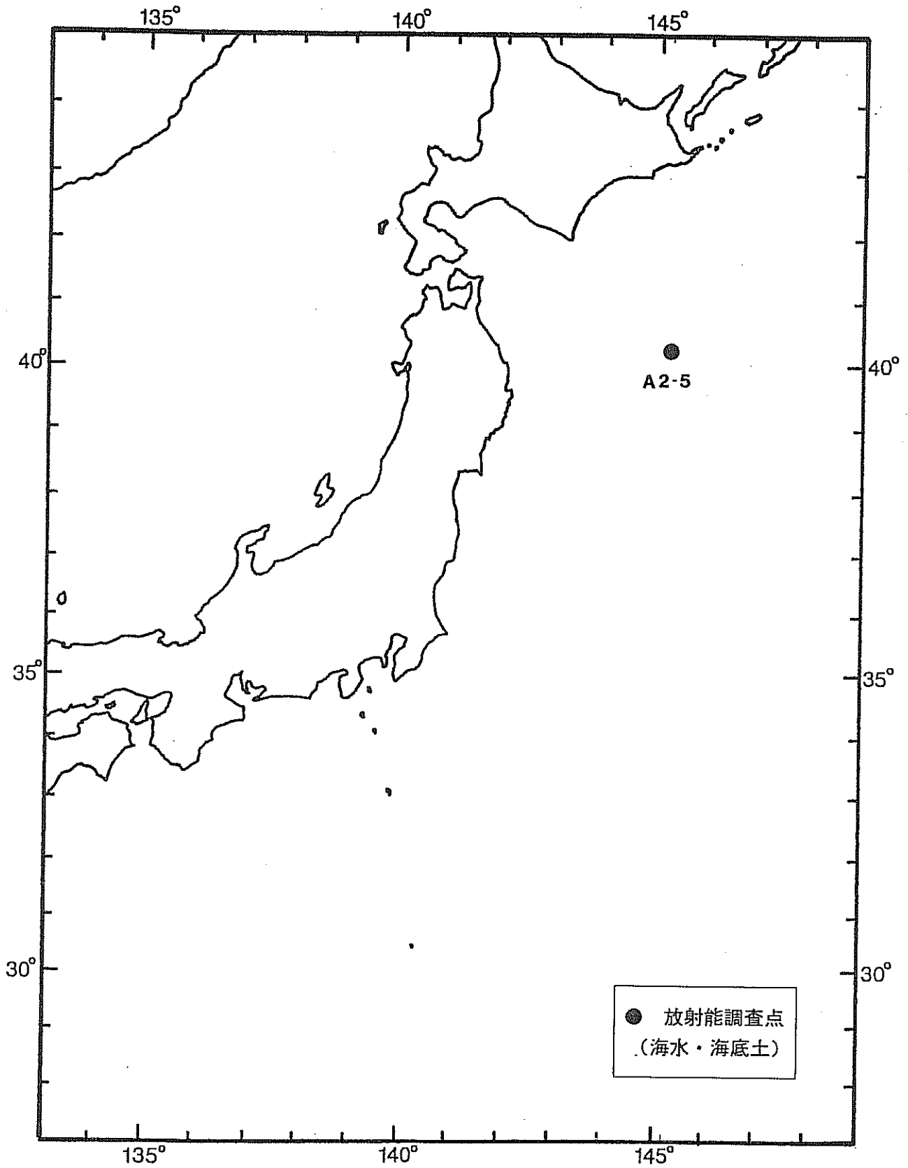
図3-1 北太平洋西部海域における放射能調査の試料採取点
