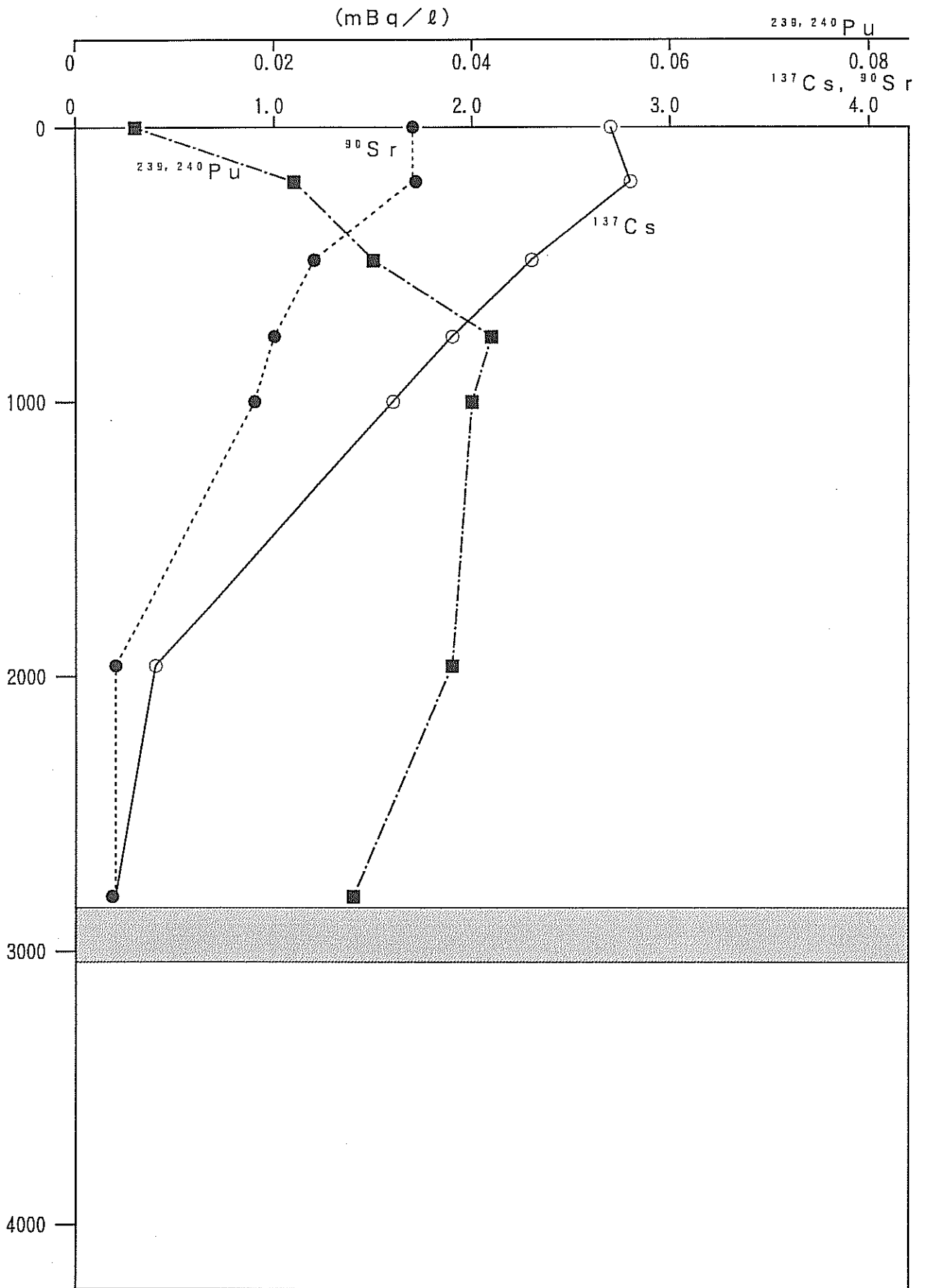
図3-6 測点 NO-3 における海水中の Pu-239,240、Cs-137 及び Sr-90 の鉛直分布
