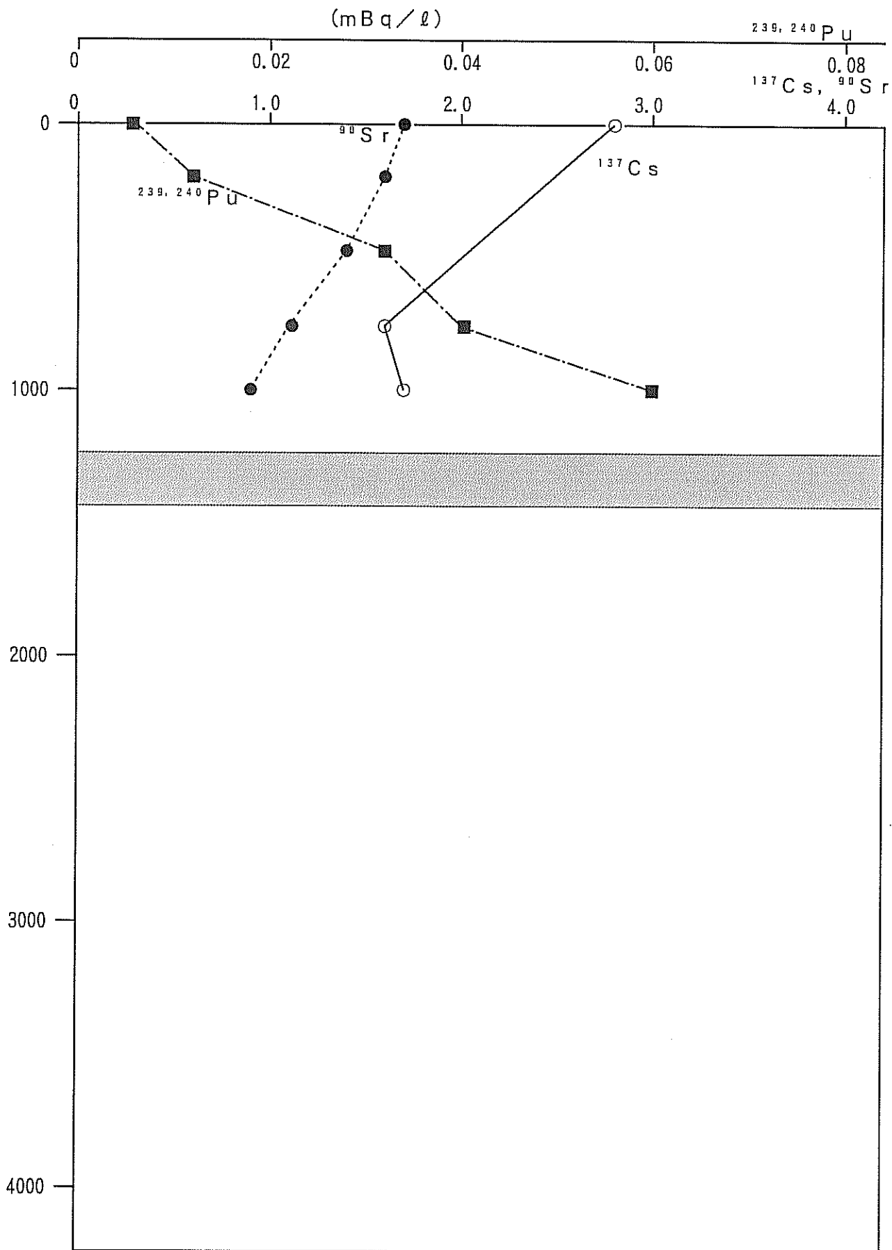
図3-7 測点NO-4における海水中のPu-239,240、Cs-137及びSr-90の鉛直分布
