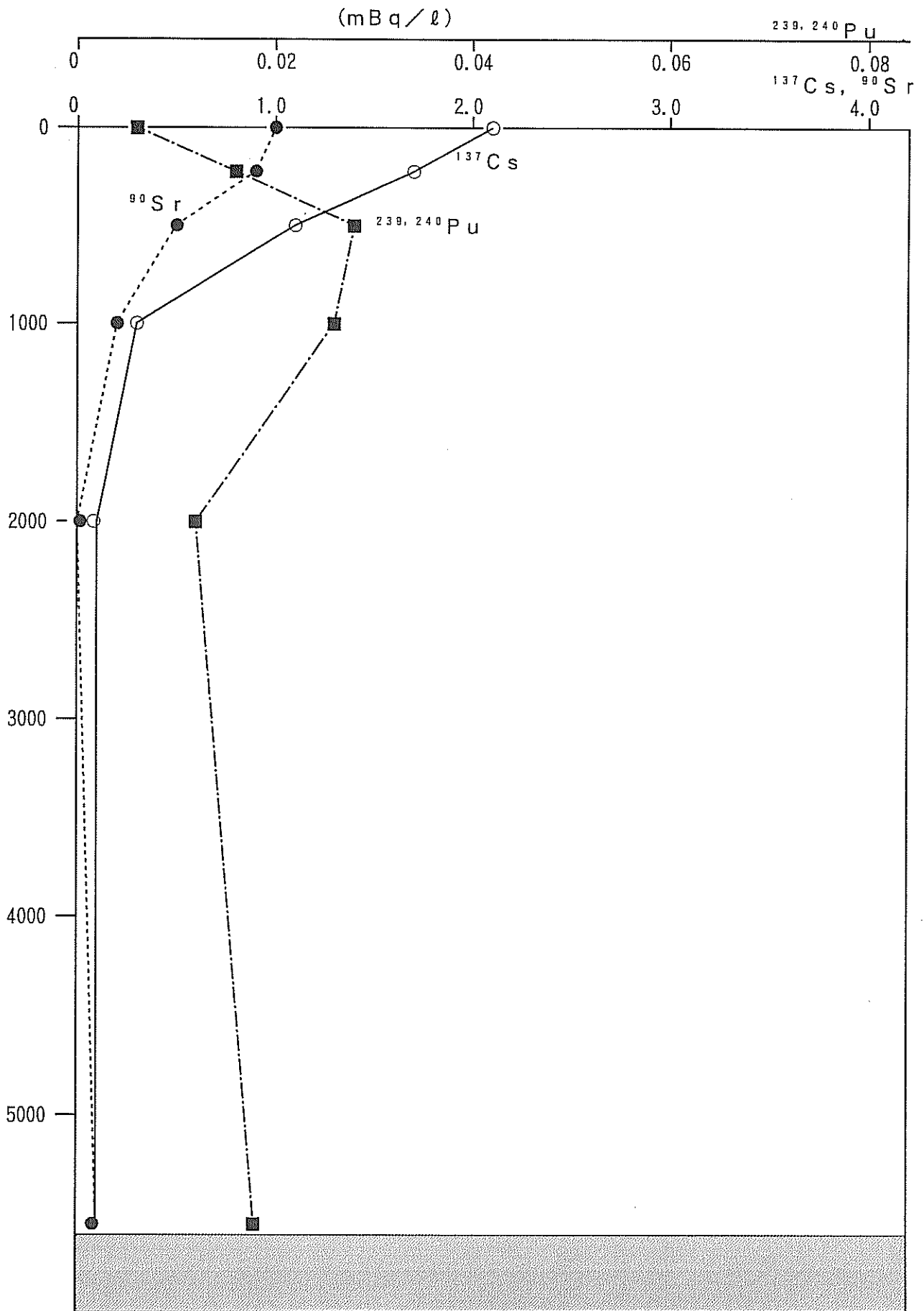
図 3 - 2 測点 A 2-5 における海水中の Pu-239,240、Cs-137 及び Sr-90 の鉛直分布
