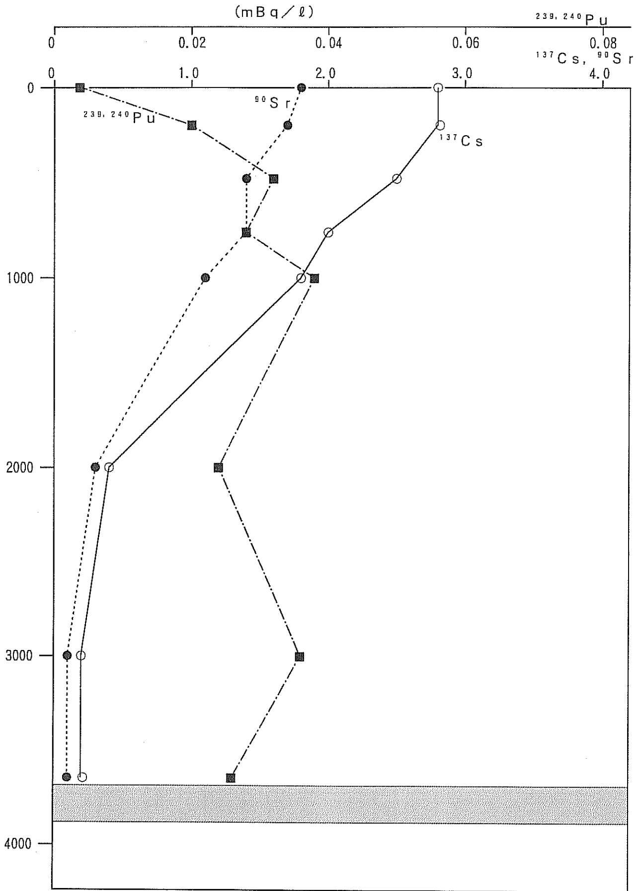
図3-10 測点NO-8における海水中のPu-239,240、Cs-137及びSr-90の鉛直分布
