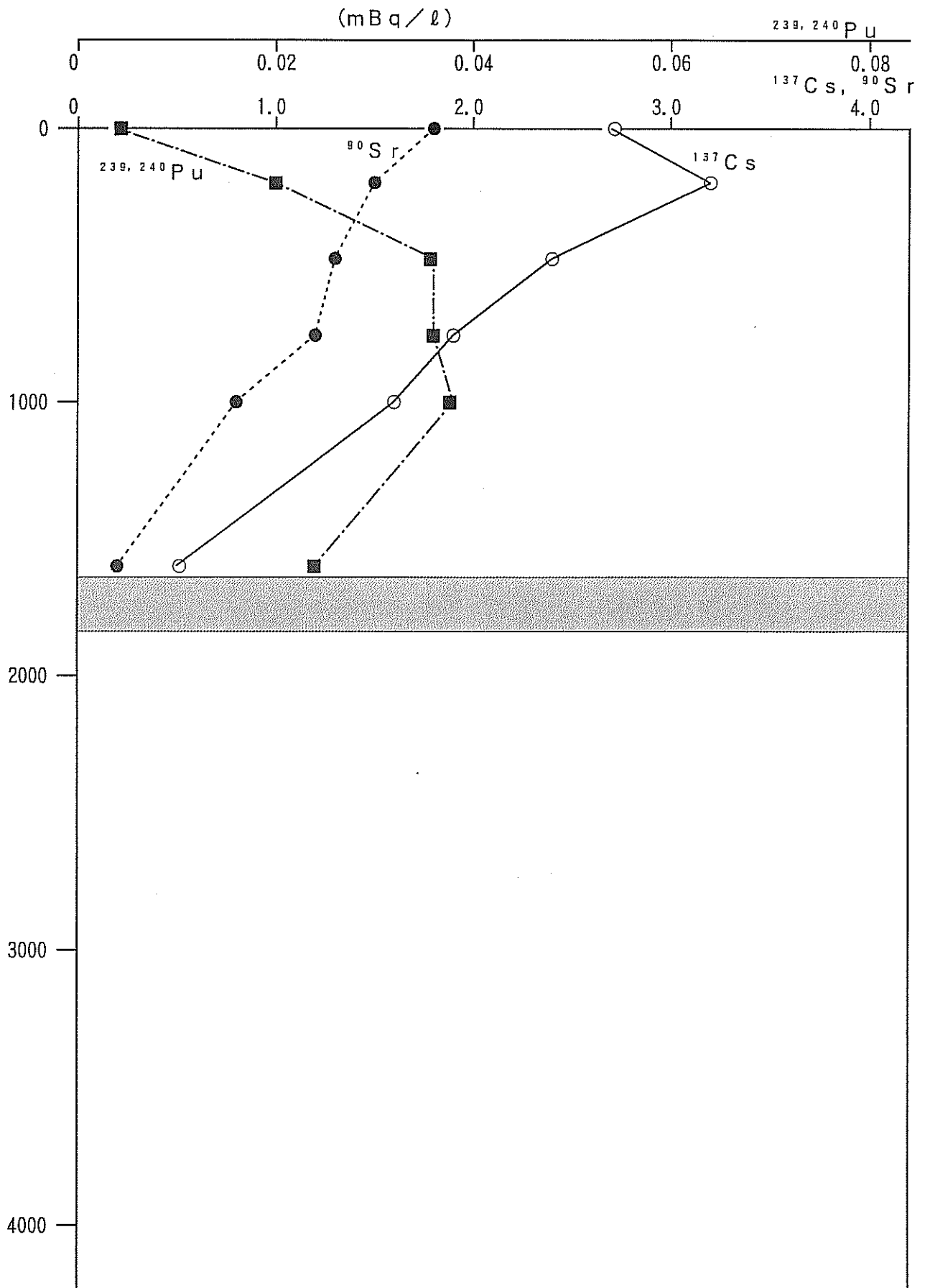
図3-5 測点NO-2における海水中のPu-239,240、Cs-137及びSr-90の鉛直分布
