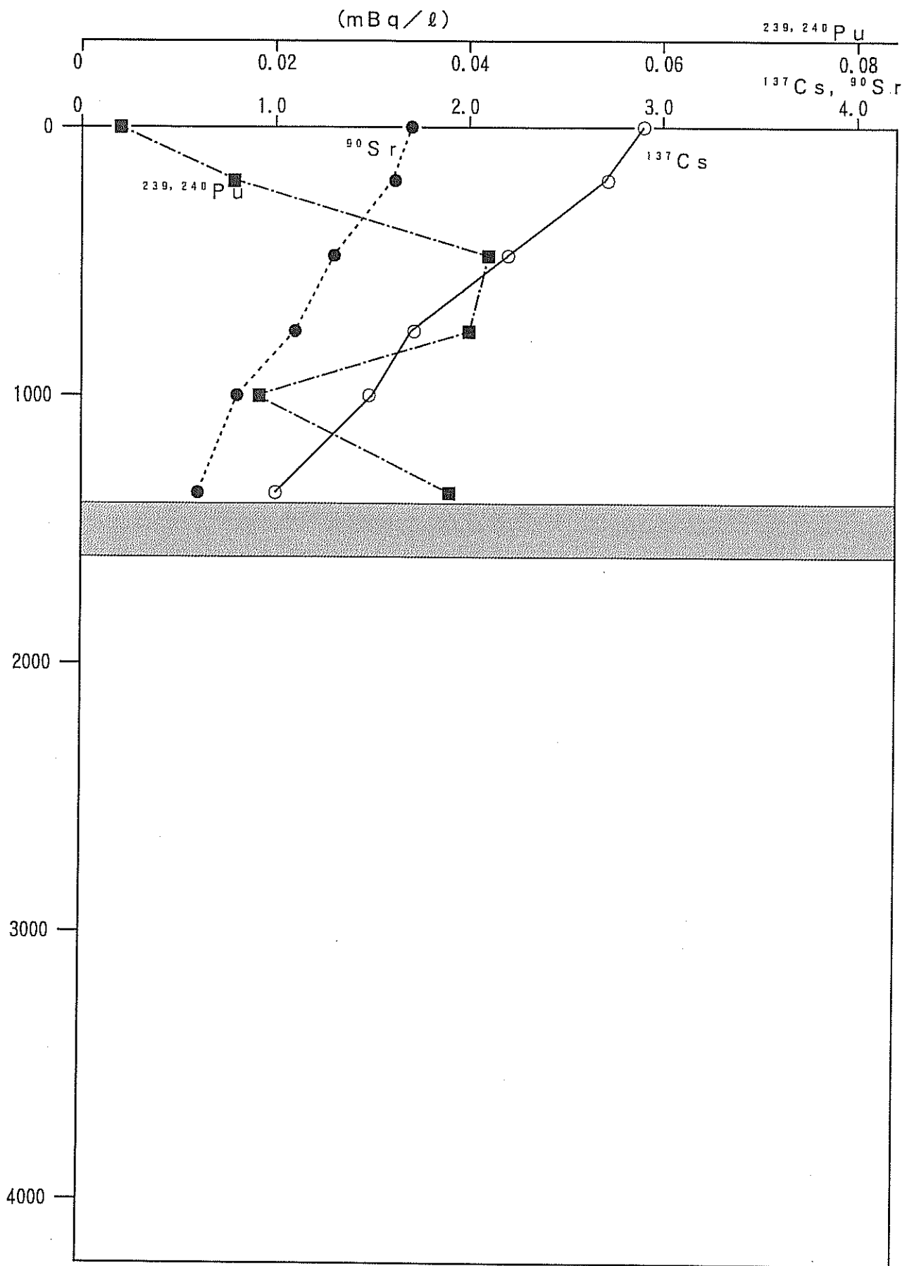
図3-8 測点NO-5における海水中のPu-239,240、Cs-137及びSr-90の鉛直分布
