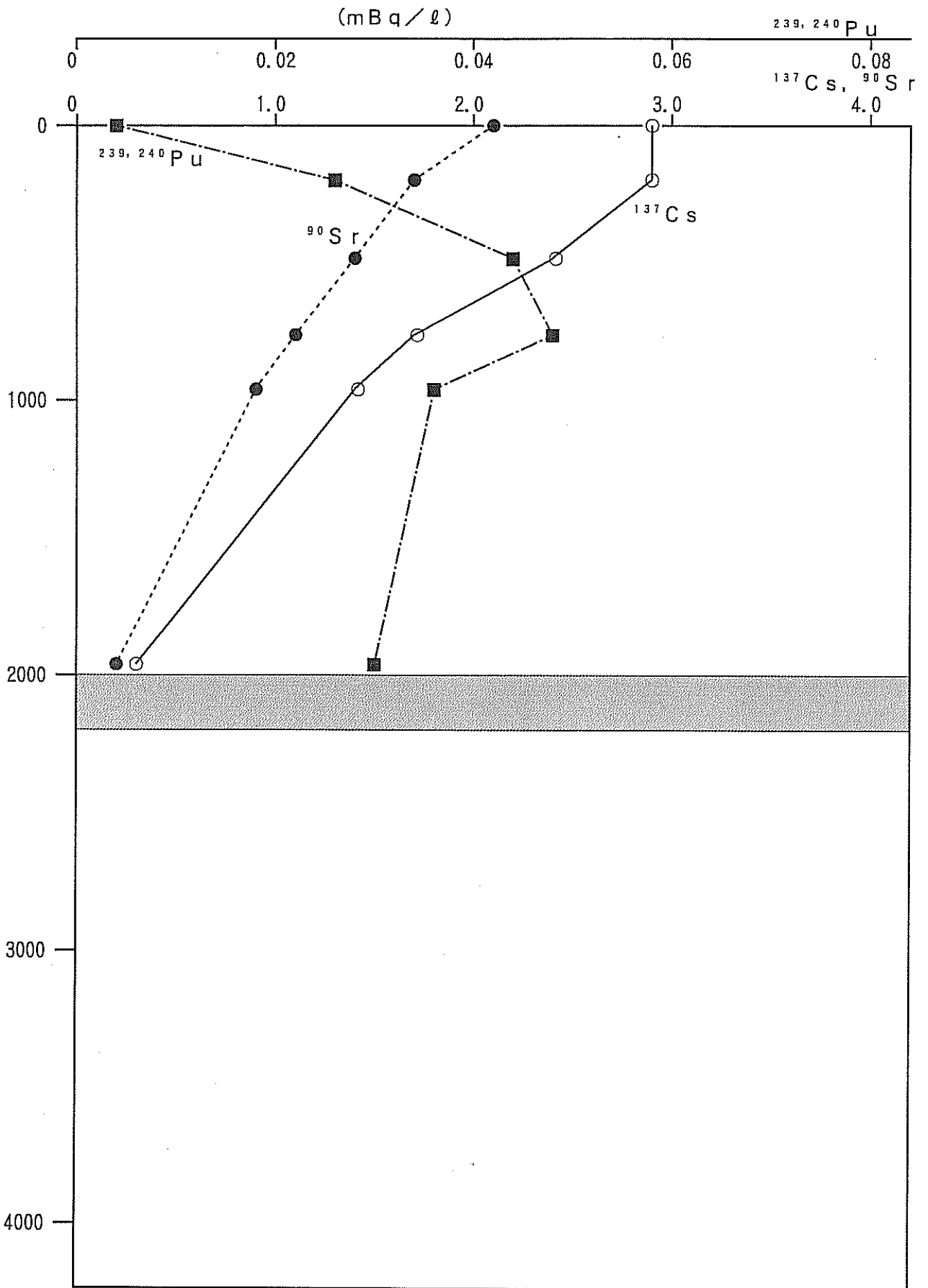
図 3-4 測点 NO-1 における海水中的の Pu-239,240、Cs-137 及び Sr-90 の鉛直分布
