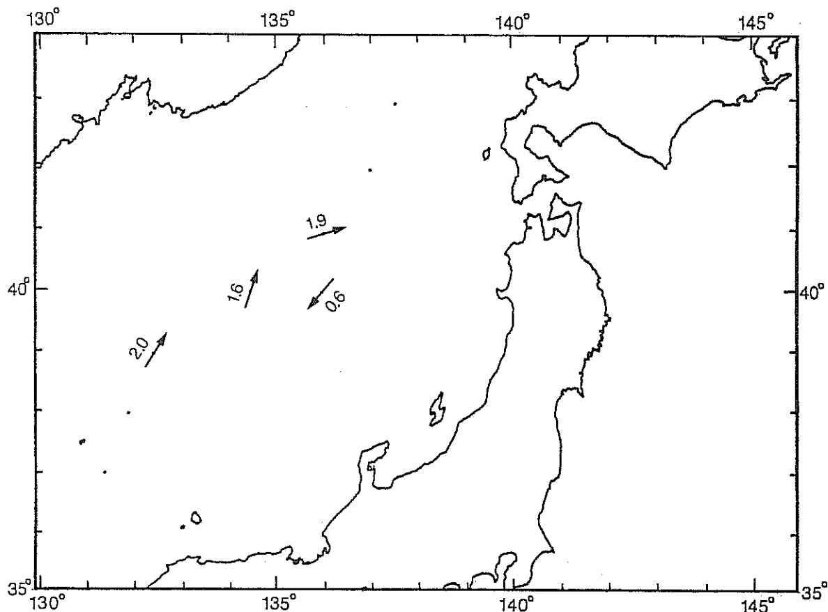
図 3 - 11 底上 100 m における平均流向流速図 (単位 ; cm/sec)
