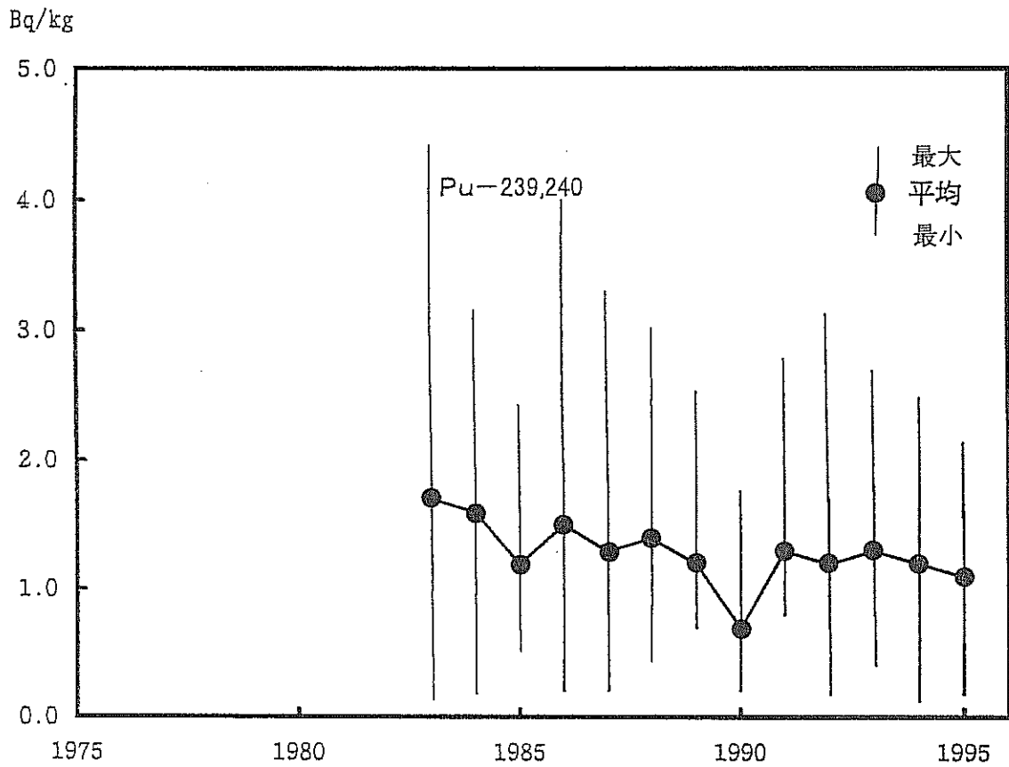
図 1 - 3 日本近海海底土中の Pu-239、240 の経年変化
