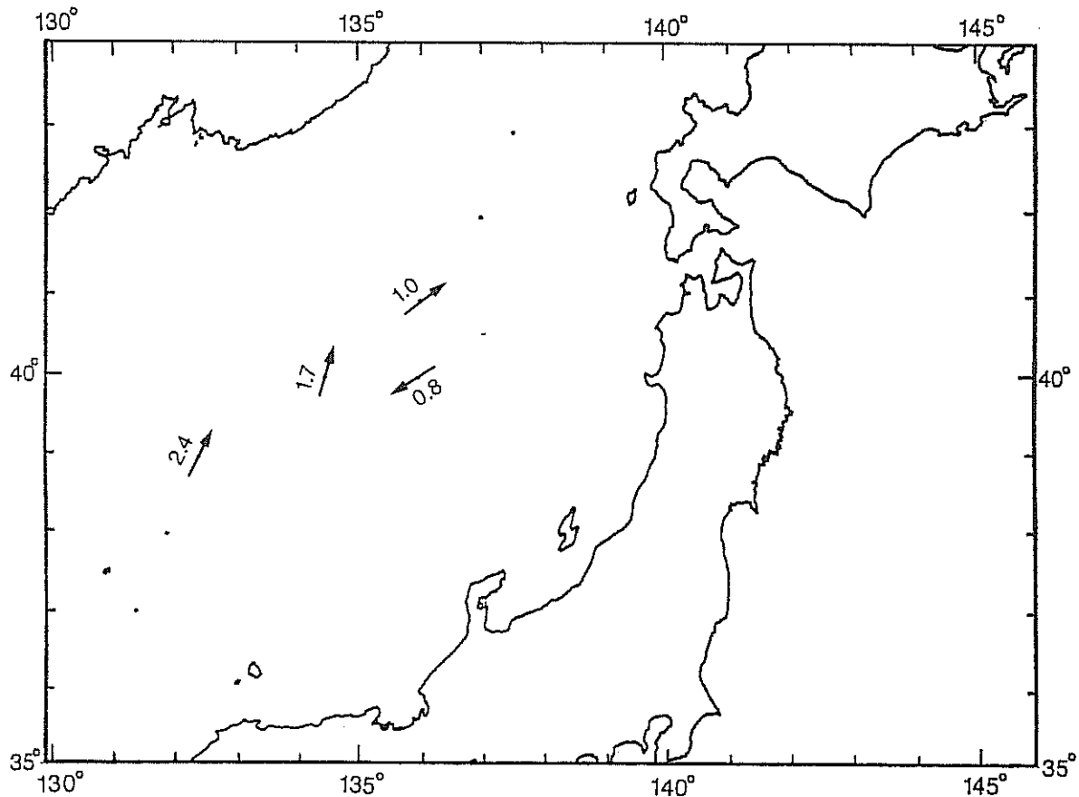
図 3 - 12 底上 50 m における平均流向流速図 (単位 ; cm/sec)
