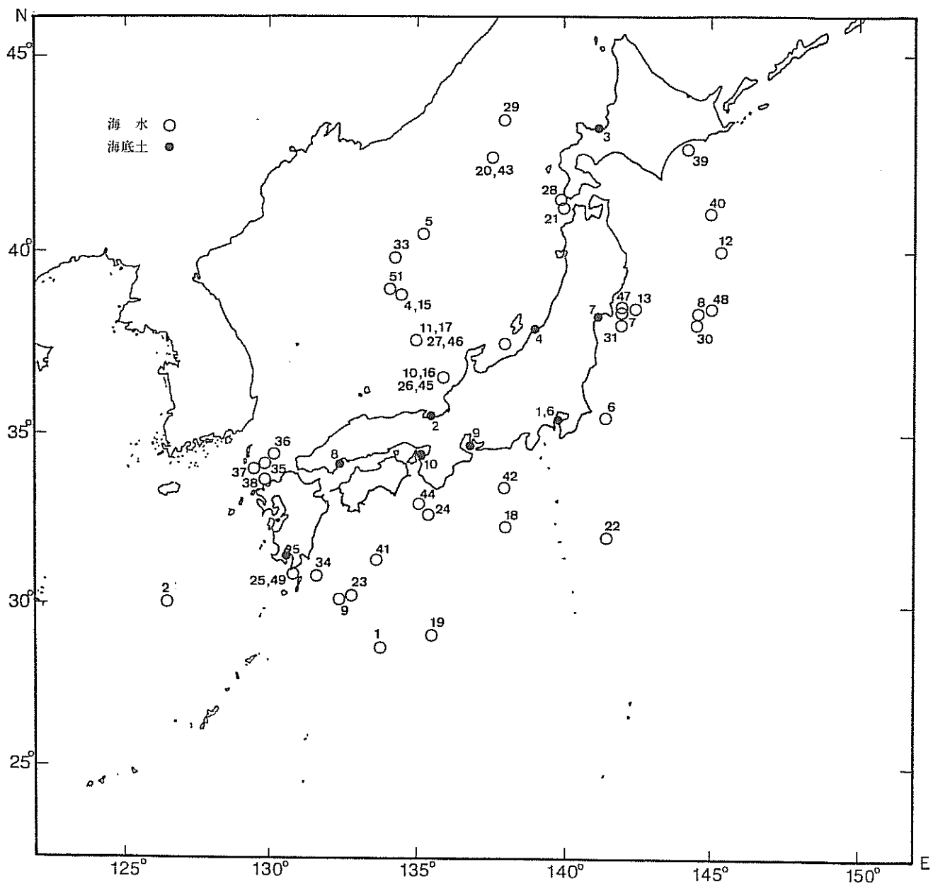
図 1 - 1 日本近海放射能調査の試料採取点及び試料番号 (平成 4 年)
