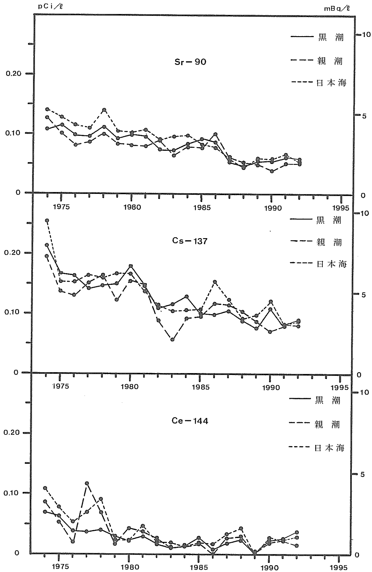
図1-2 日本近海表面海水中的 Sr-90、Cs-137及び Ce-144の年平均濃度の経年変化
