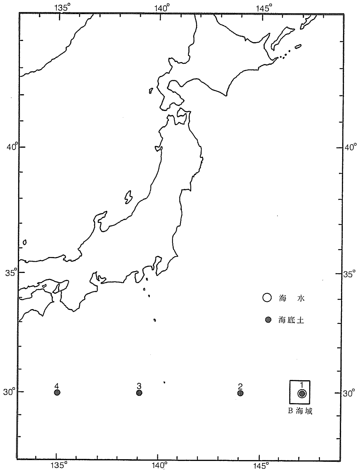
図 3 - 1 北太平洋西部海域放射能調査の試料採取点及び測点番号
