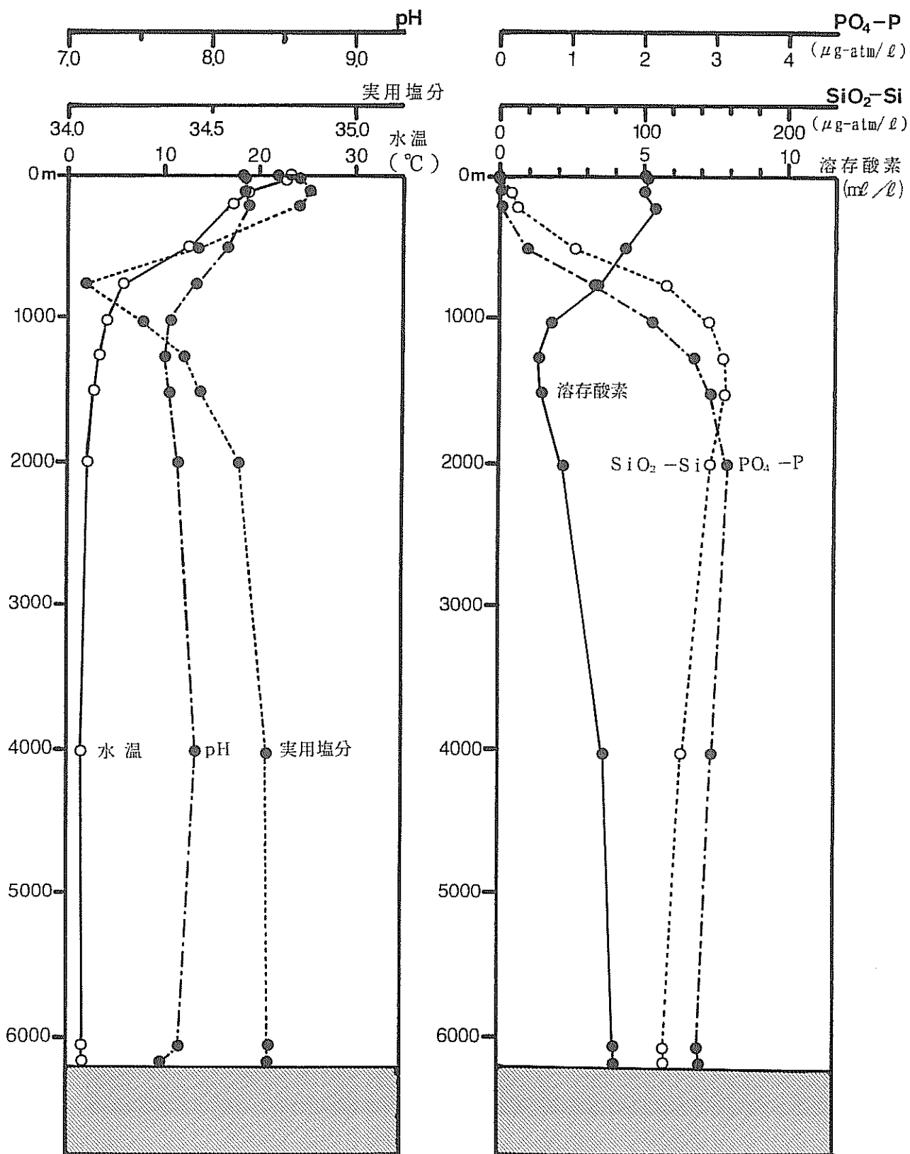
図3-3 測点1 (30°00'N, 147°00'E) における海水中の水温、実用塩分、溶存酸素、pH、りん酸塩( \text{PO}_4\text{-P} )及びけい酸塩( \text{SiO}_2\text{-Si} )の鉛直分布
