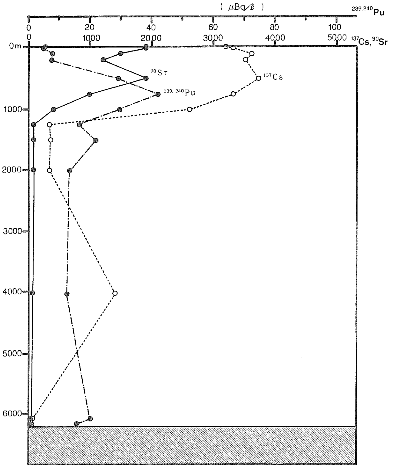
図 3—2 測点 1 (30°00'N, 147°00'E) における海水中の Pu-239,240、Cs-137及び Sr-90 の鉛直分布
