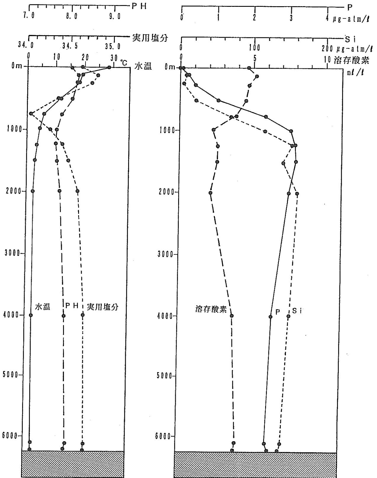
図3-3 測点3 (30°00'N, 147°00'E) における海水中の水溫、実用塩分、溶存酸素、pH、りん酸塩(P)及びけい酸塩(Si)の鉛直分布
