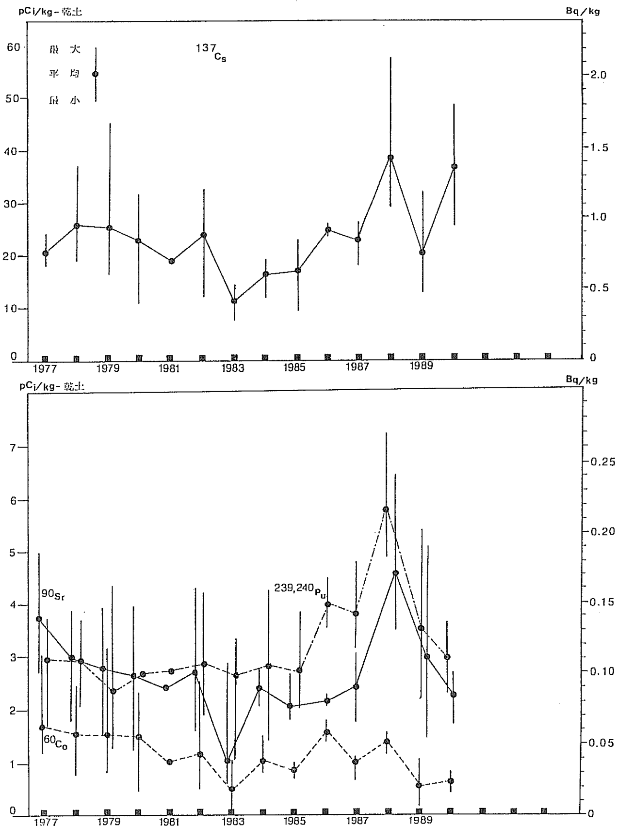
図3-6 放射性固化体の試験的海洋処分候補海域 (B 海域) における海底土中の Pu-239, 240、Cs-137及び Co-60の経年変化
