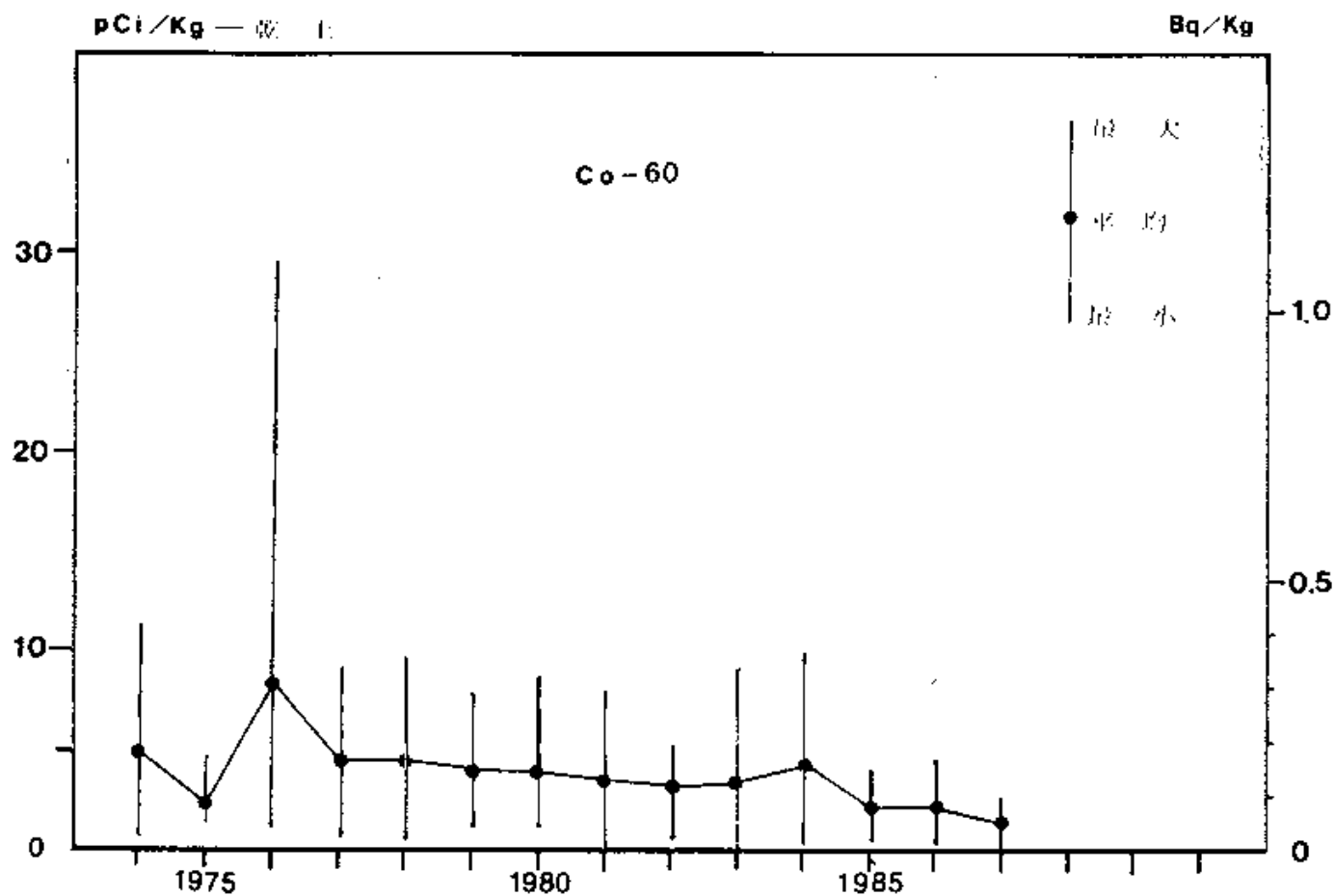
図 1-7 日本近海海底土中の Co-60 の経年変化
