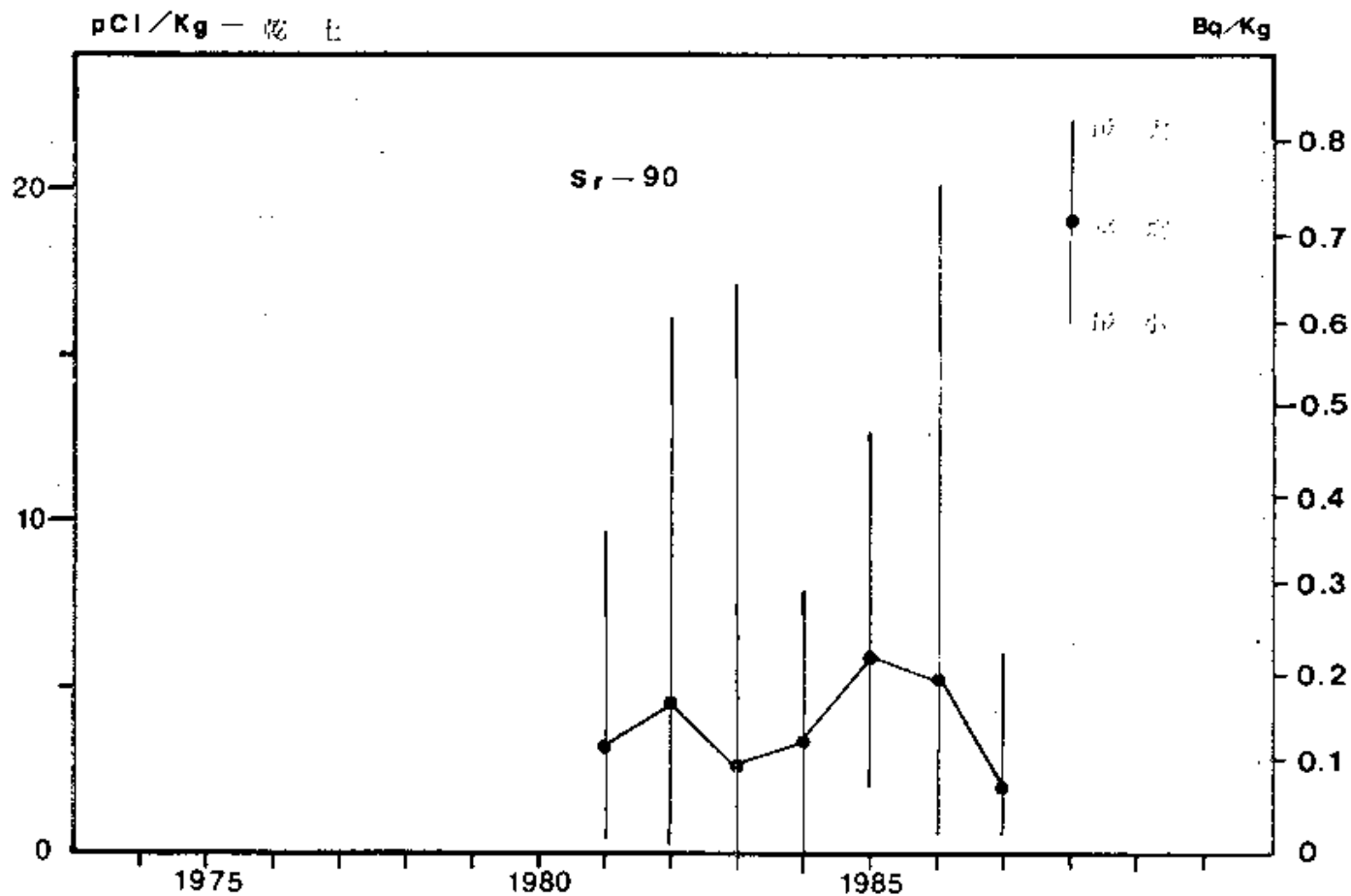
図 1-6 日本近海海底土中の Sr-90 の経年変化
