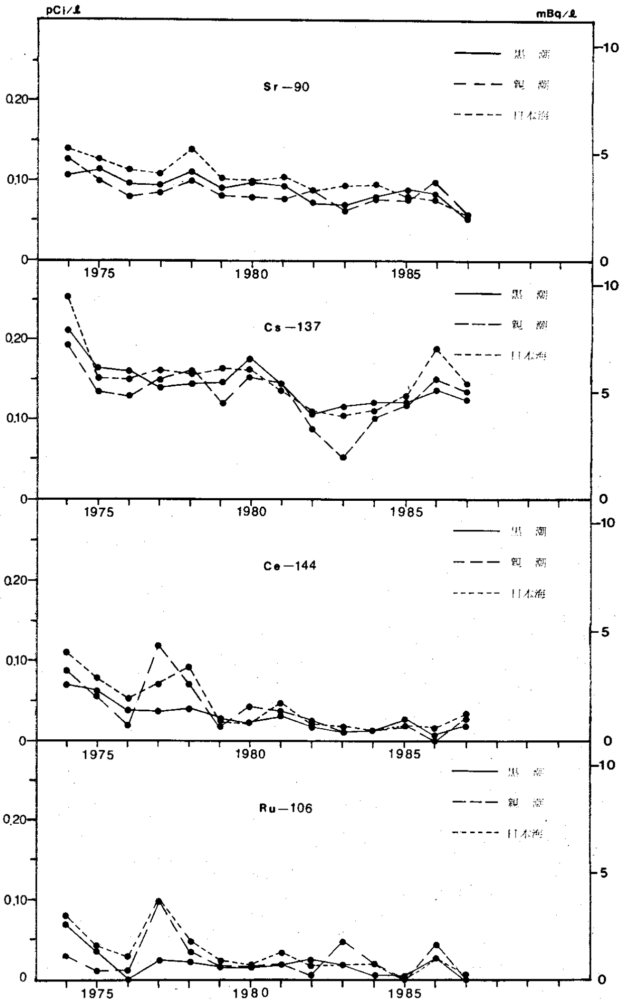
図1-2 日本近海表面海水中のSr-90、Cs-137、Ce-144及びRu-106の年平均濃度の経年変化
