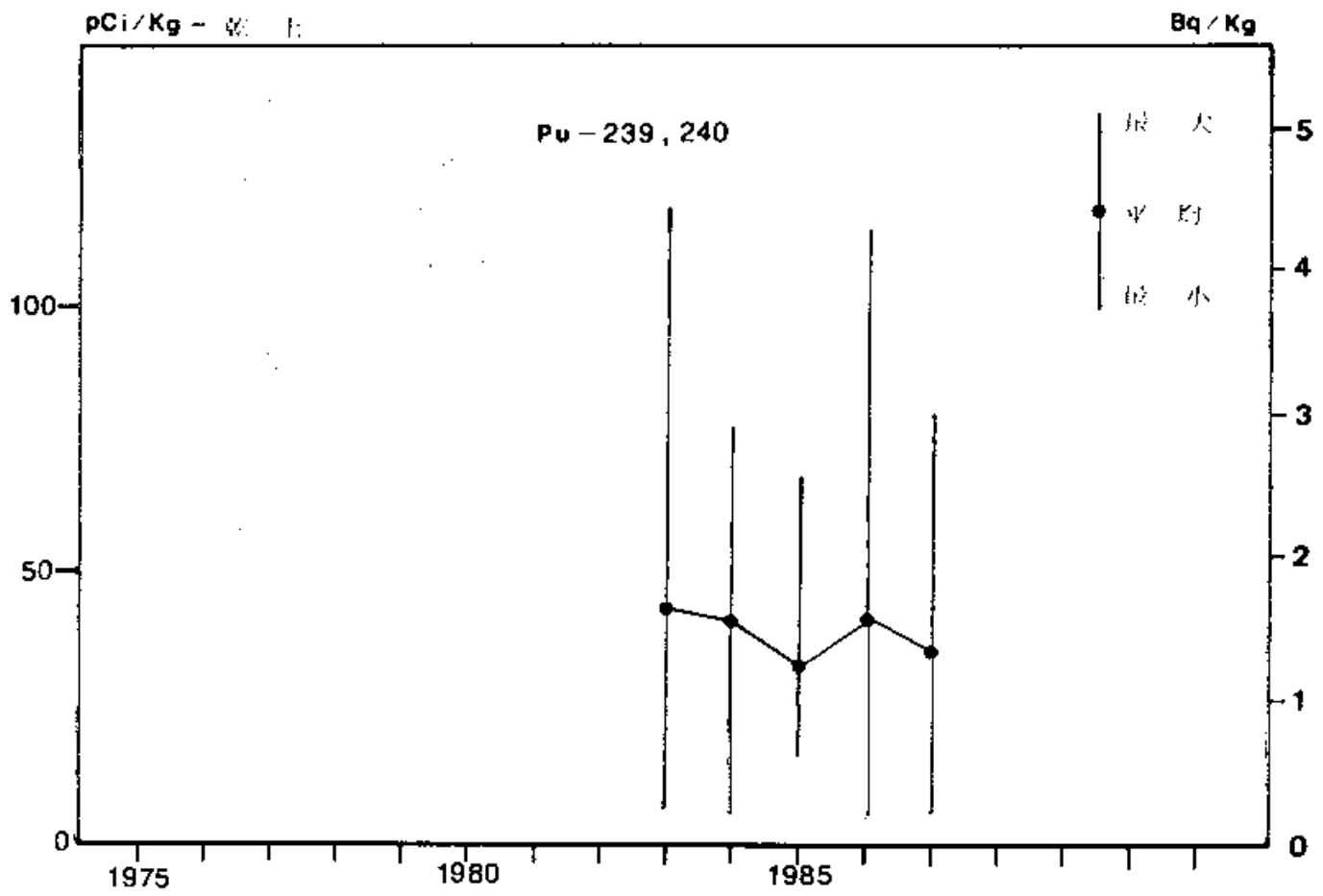
図1-4 日本近海海底土中のPu-239, 240の経年変化
