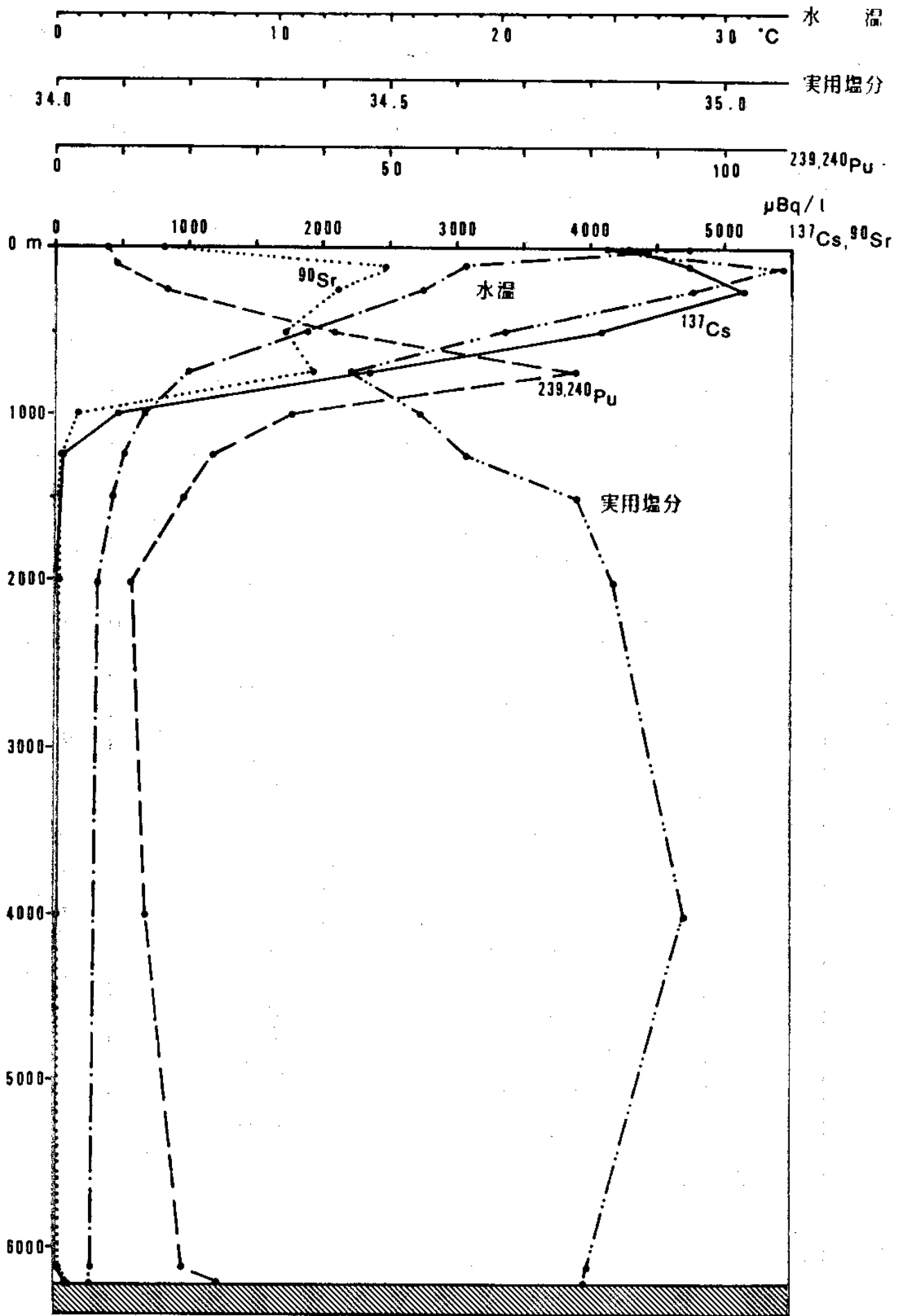
図3-2 測点4 (30°01' N, 146°58' E) における海水中の Pu-239, 240、Cs-137、Sr-90 及び水温、塩分の鉛直分布
