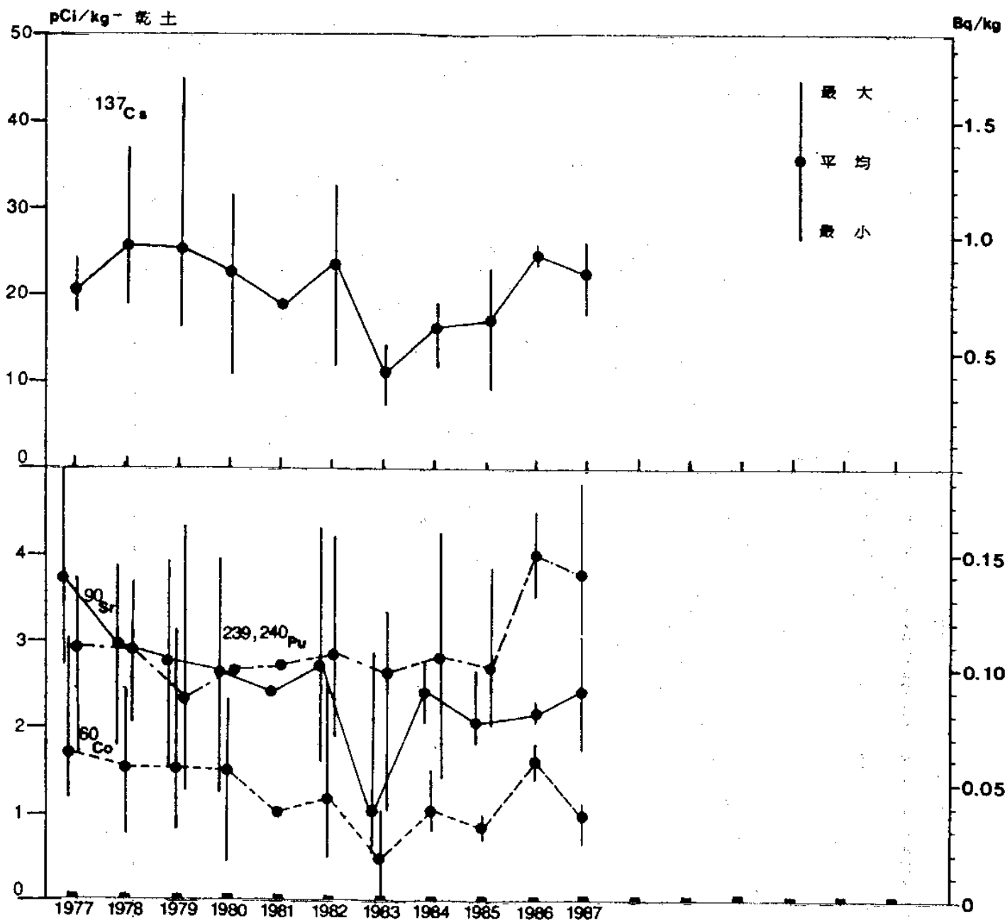
図 3-4 放射性固化体の試験的海洋処分候補海域 (B 海域) における海底土中の Pu-239, 240、Cs-137、Sr-90 及び Co-60 の経年変化
