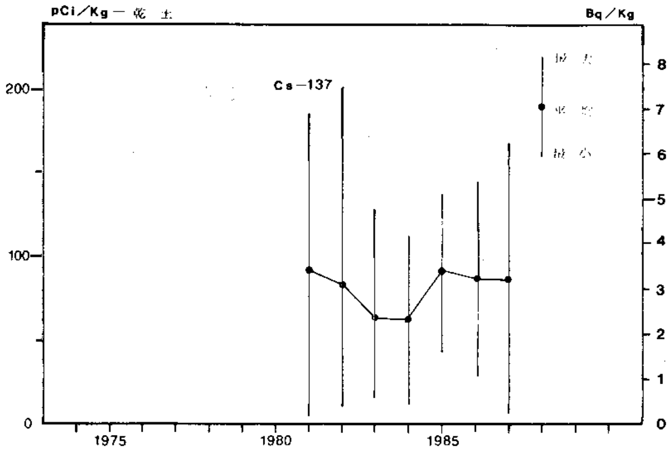
図1-5 日本近海海底土中のCs-137の経年変化
