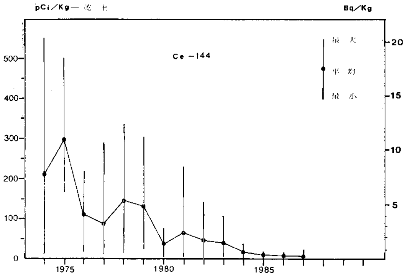
図 1-9 日本近海海底土中のCe-144の経年変化
