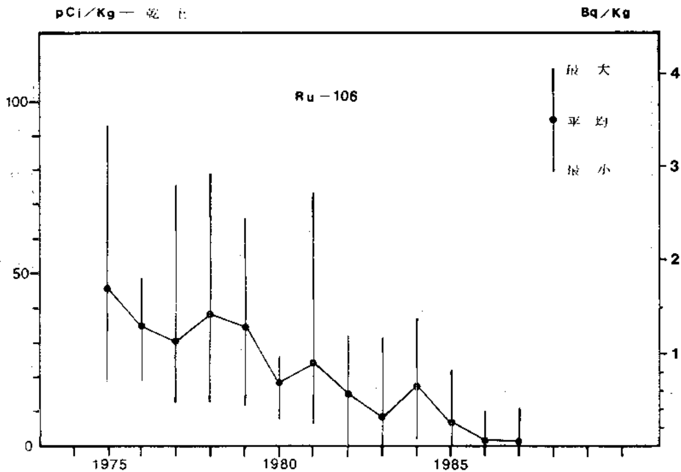
図 1-8 日本近海海底土中のRu-106の経年変化
