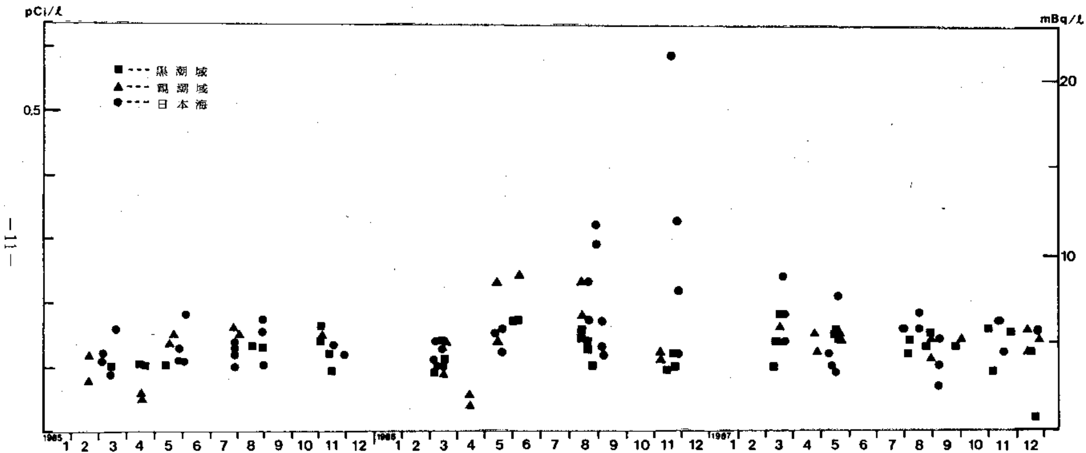
図 1-3 1985～1987年における表面海水中的Cs-137の経年変化
