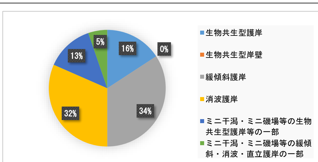
図 B3-2 東京湾における生物共生型港湾構造物の箇所数割合
