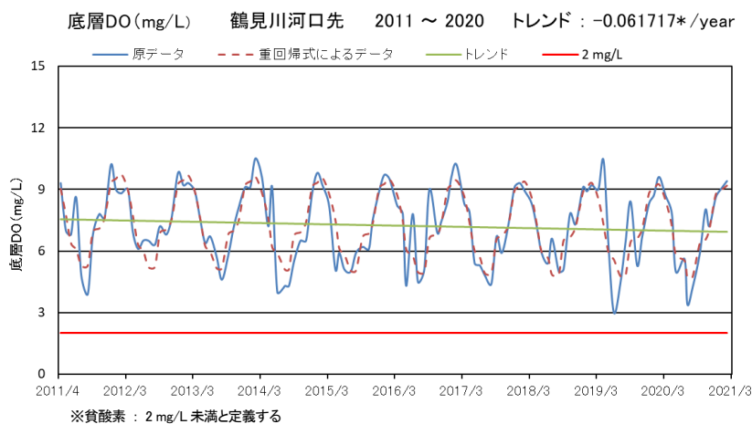
図 B4-4 DO (底層) (mg/L) の時系列変化および重回帰分析結果 (鶴見川河口先)
