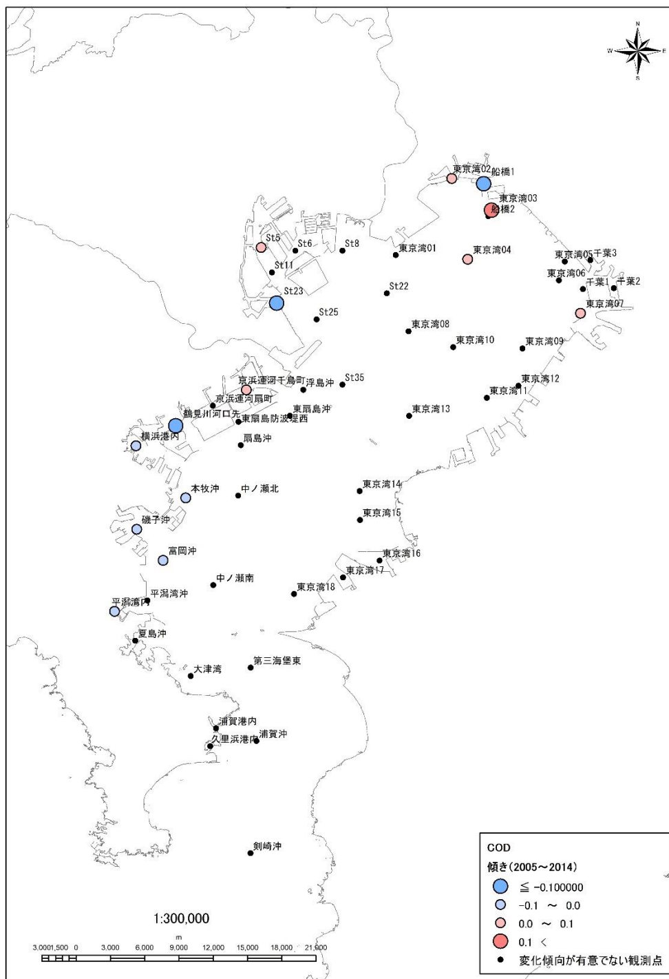
図 A2-6 CODの上昇地点および改善地点の空間分布 (2014年度)
