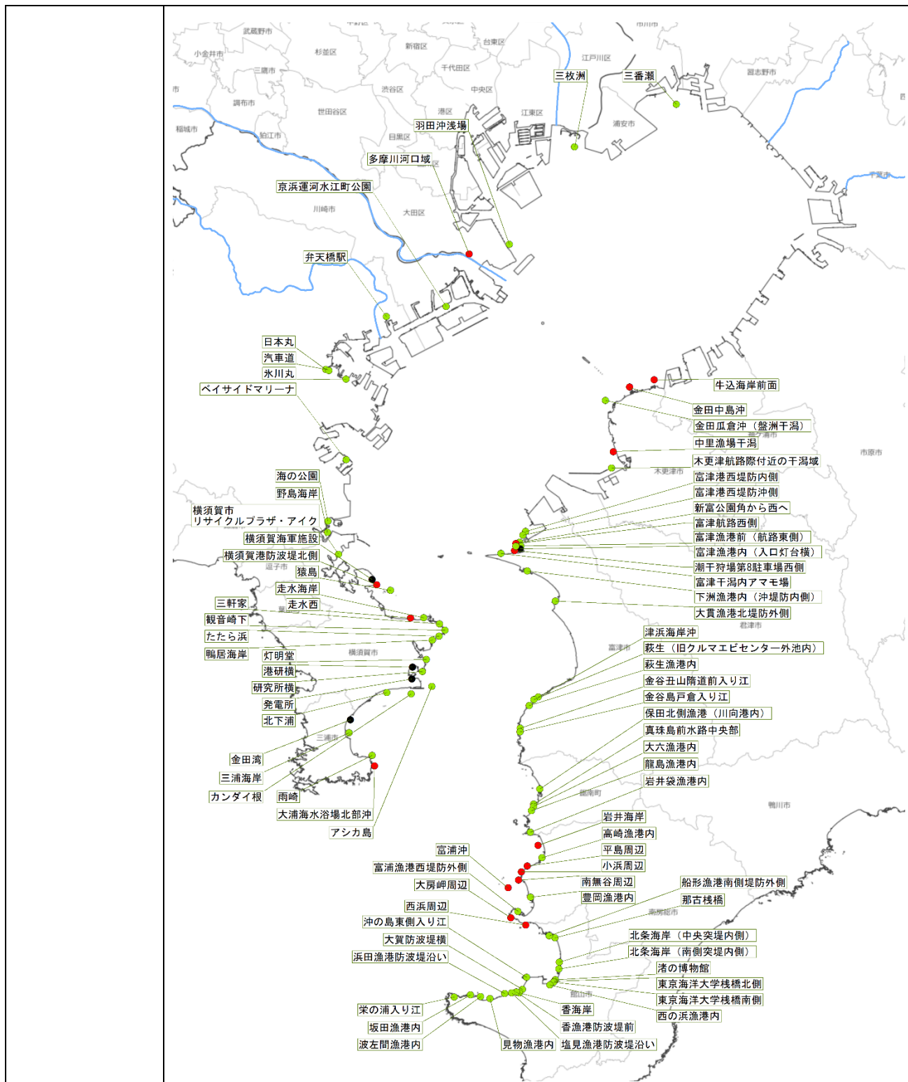
図 B2-2 東京湾における藻場の分布 (平成 27 年度集計から、17 箇所増加 (図の●)、5 箇所減少 (図の●))
