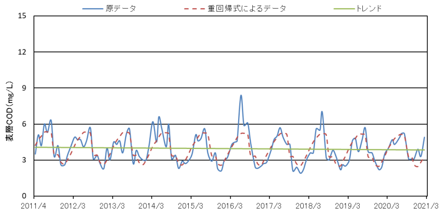
図 A2-2 COD (mg/L) の時系列変化および重回帰分析結果（鶴見川河口先）
