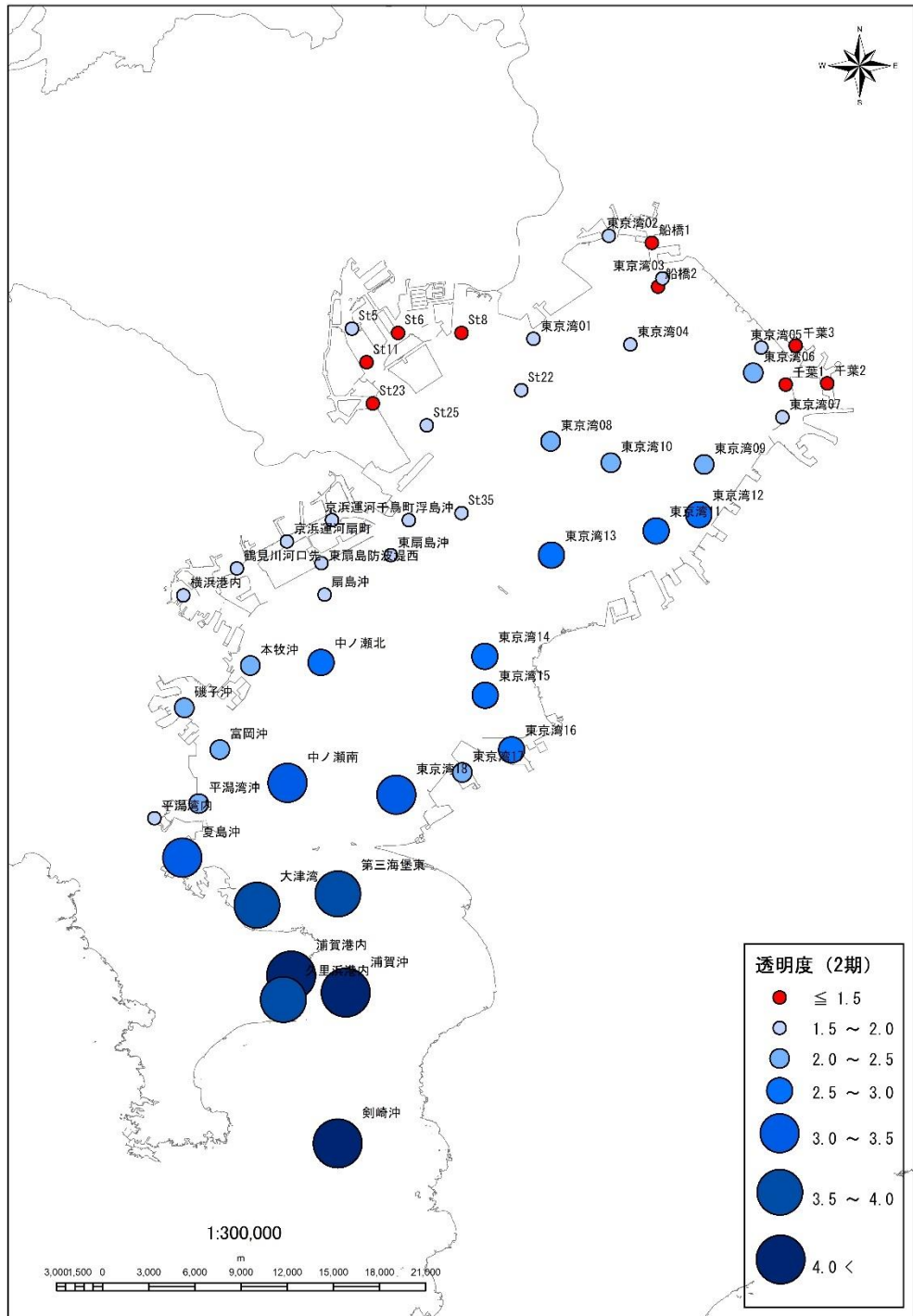
図 A1-12 夏季透明度の期間平均値 (第二期)
