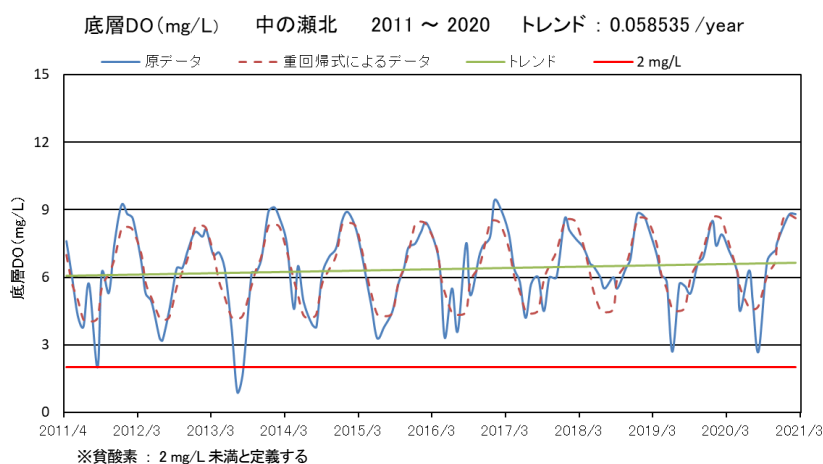
図 B4-5 DO (底層) (mg/L) の時系列変化および重回帰分析結果 (中ノ瀬北)
