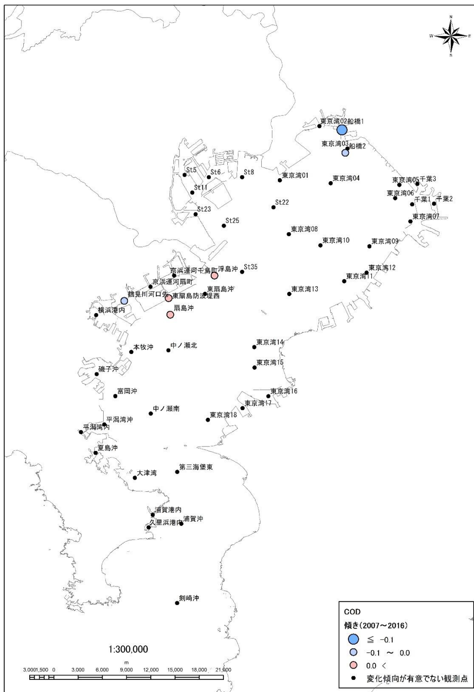
図 A2-8 CODの上昇地点および改善地点の空間分布 (2016年度)
