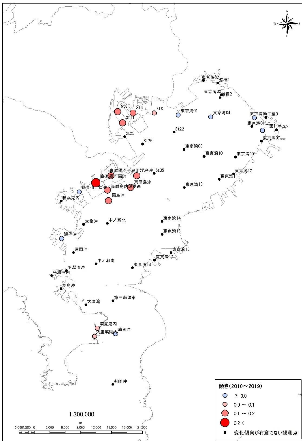
図 A2-11 CODの上昇地点および改善地点の空間分布 (2019 年度)
