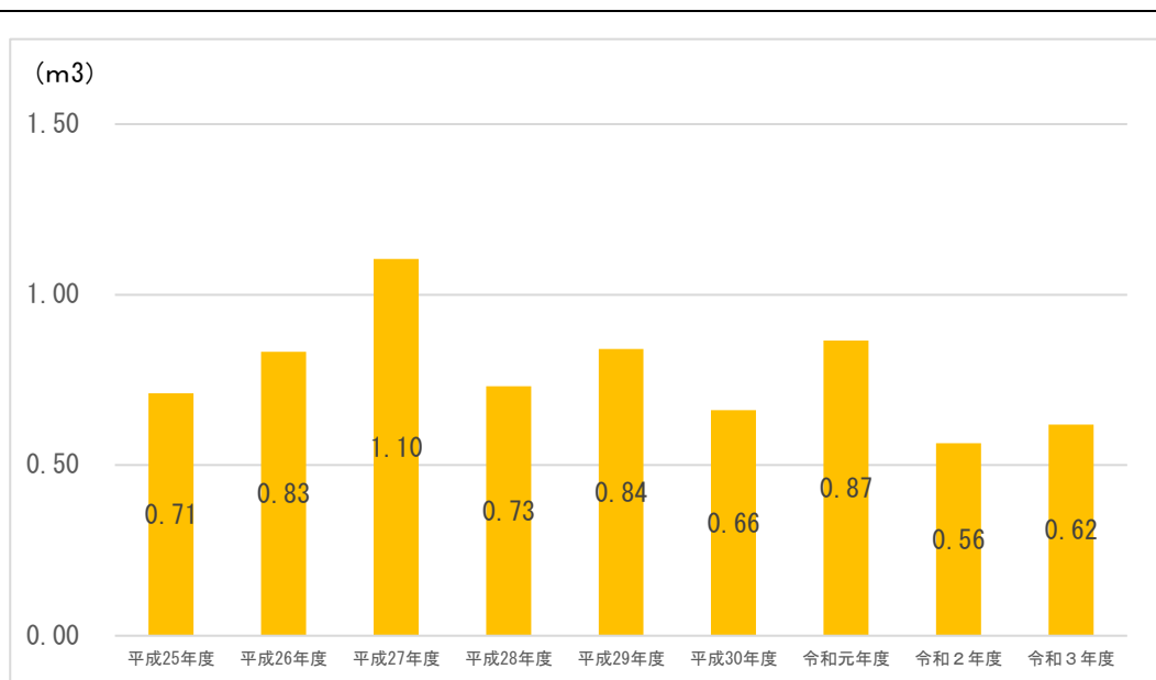
図 A5-1 東京湾における 1ha あたりのゴミ回収量 (参考)
