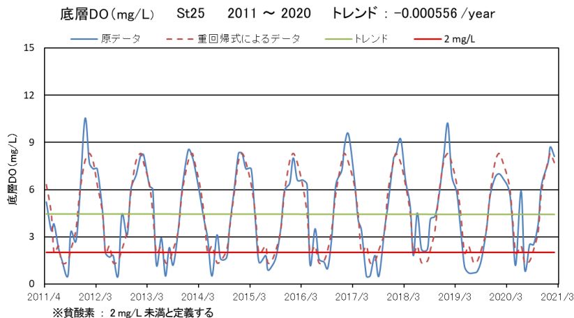
図 B4-3 DO (底層) (mg/L) の時系列変化および重回帰分析結果 (St. 25)
