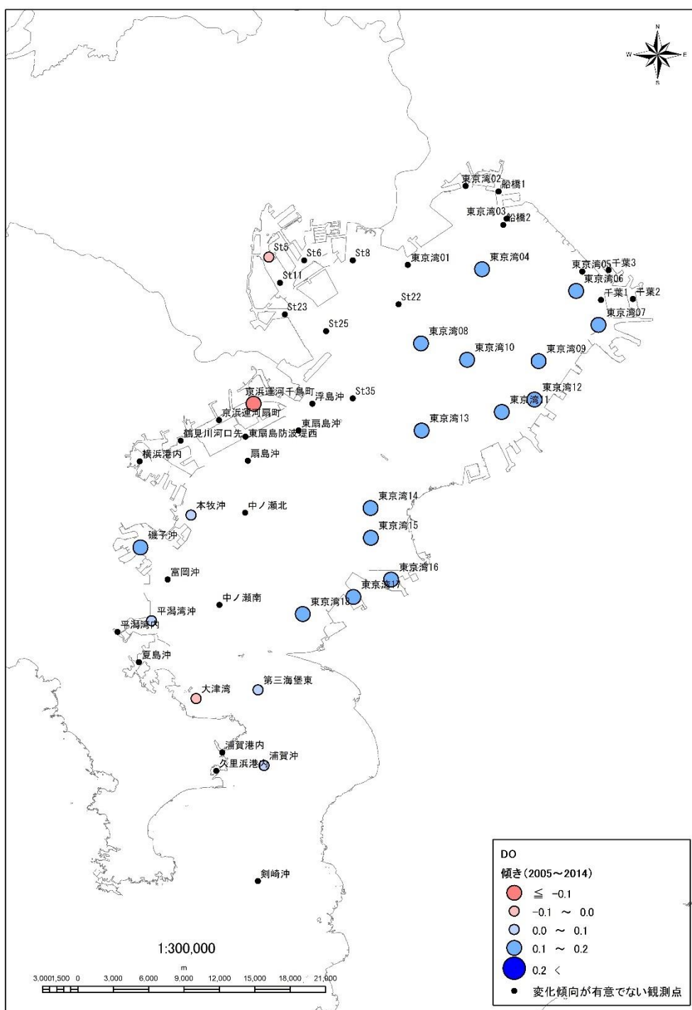
図 B4-7 DO (底層) の上昇・低下地点の空間分布 (2014 年度 : 2005 年度~2014 年度)
