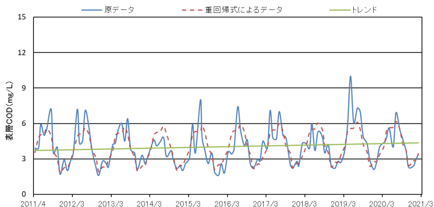
図 A2-3 COD (mg/L) の時系列変化および重回帰分析結果（ST. 25）
