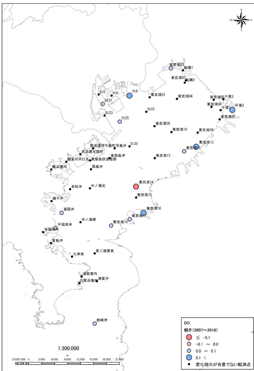
図 B4-9 DO (底層) の上昇・低下地点の空間分布 (2016 年度 : 2007 年度~2016 年度)
