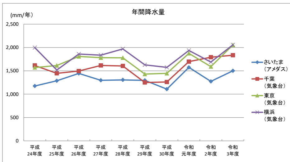
図 A3-4 年間降水量の推移
