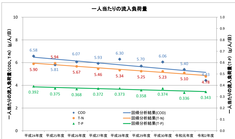
図 D6-5 一人当たりの流入負荷量の回帰分析結果
