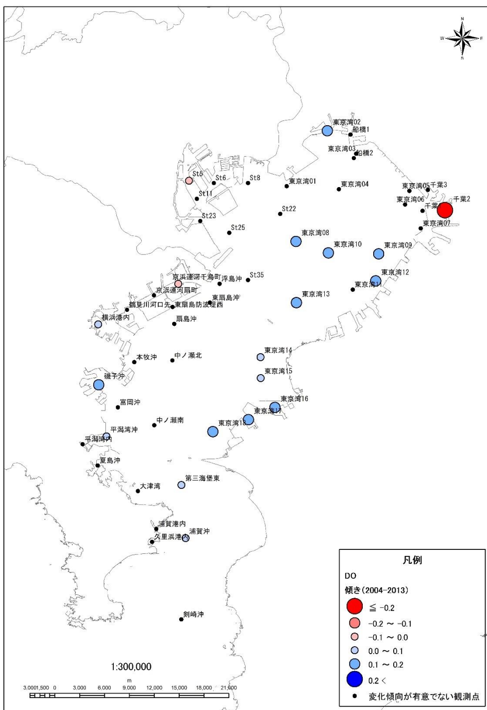
図 B4-6 DO (底層) の上昇・低下地点の空間分布 (2013 年度 : 2004 年度~2013 年度)
