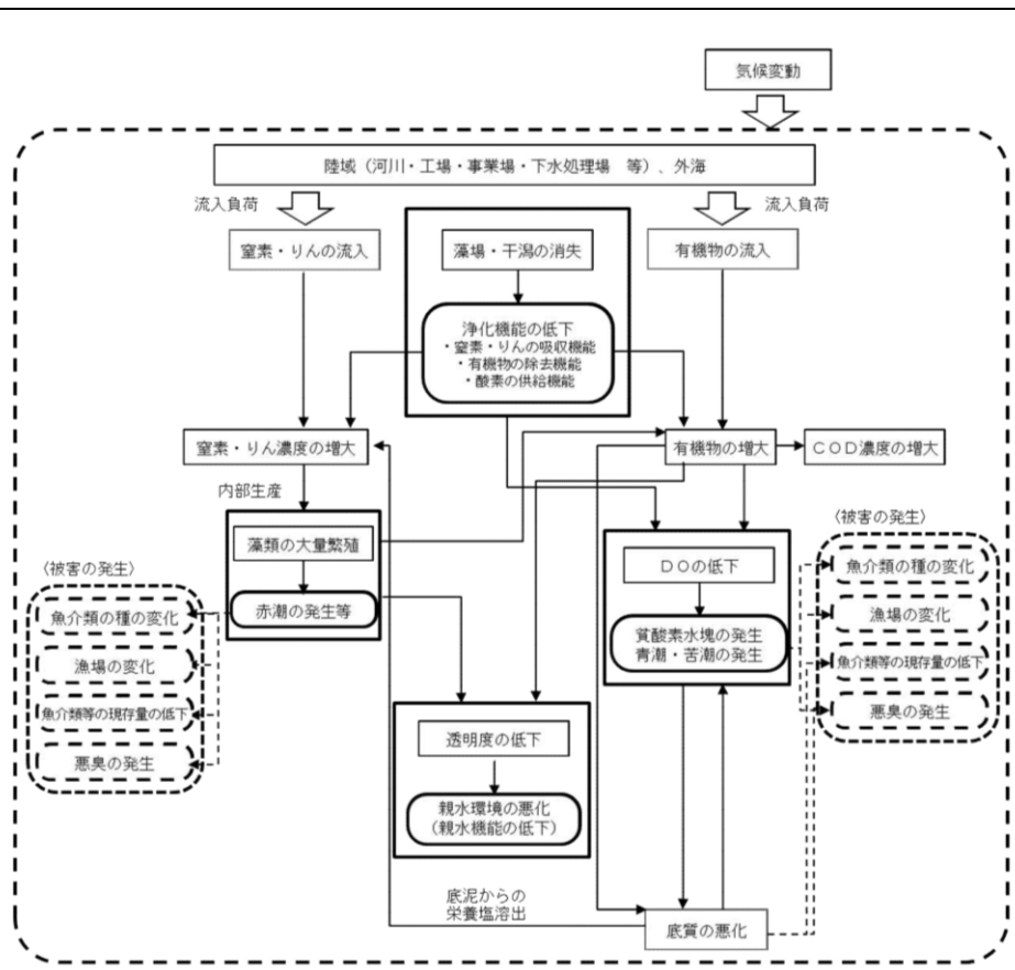
図 A1-14 閉鎖性海域における水質汚濁に影響を与える要因※ ※出典：第9次水質総量削減の在り方について（答申）（令和3年3月）
