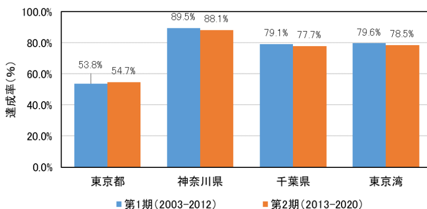
図 A1-10 第 I 期と第 II 期の目標値の達成率
