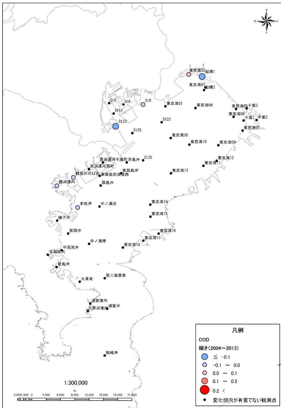
図 A2-5 CODの上昇地点および改善地点の空間分布 (2013年度)
