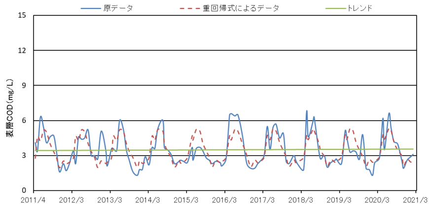
図 A2-4 COD (mg/L) の時系列変化および重回帰分析結果（東京湾 8）
