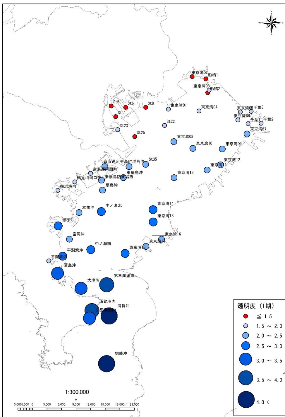
図 A1-11 夏季透明度の期間平均値 (第一期)
