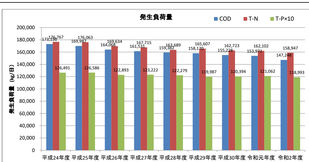
図 D6-6 一人当たりの発生負荷量
