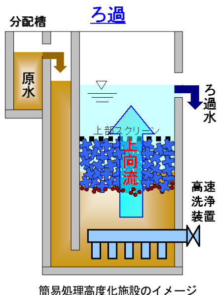
簡易処理高度化施設のイメージ
