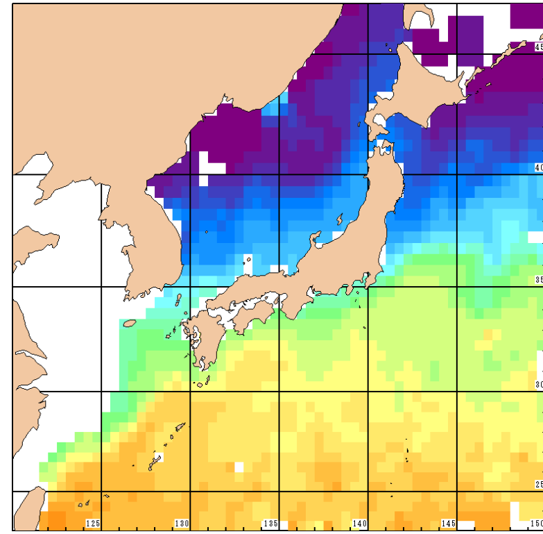
3月の水温平年値( )
