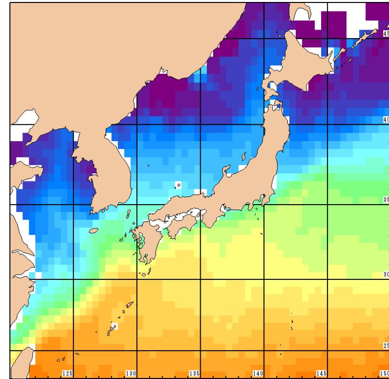
3月の水温平年値( ) 日本海洋データセンターの統計値
