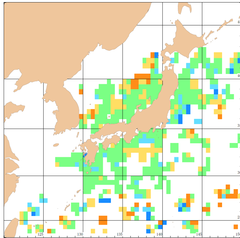
2008年3月水温平年差
