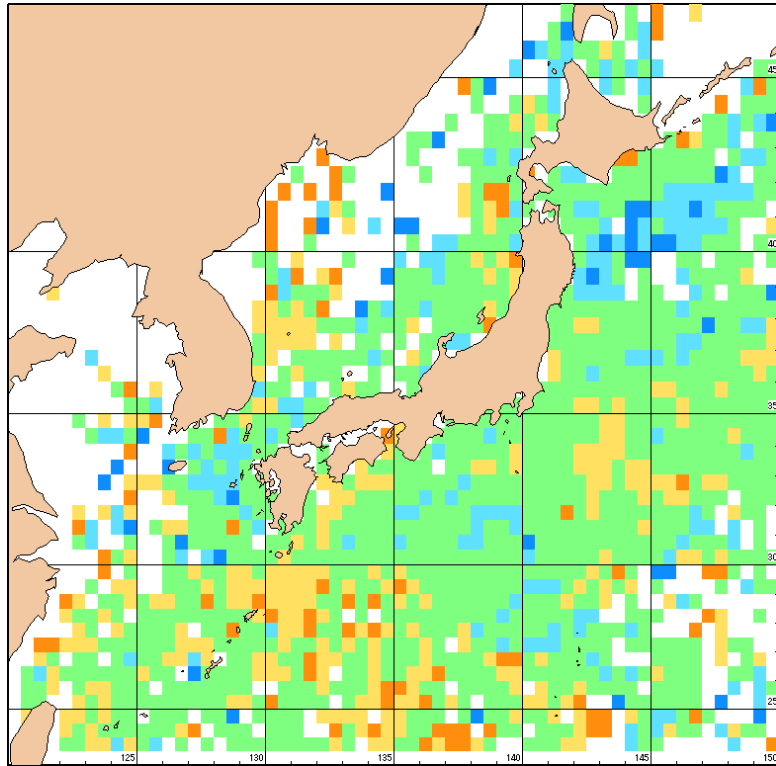
2006年5月水温平年差
