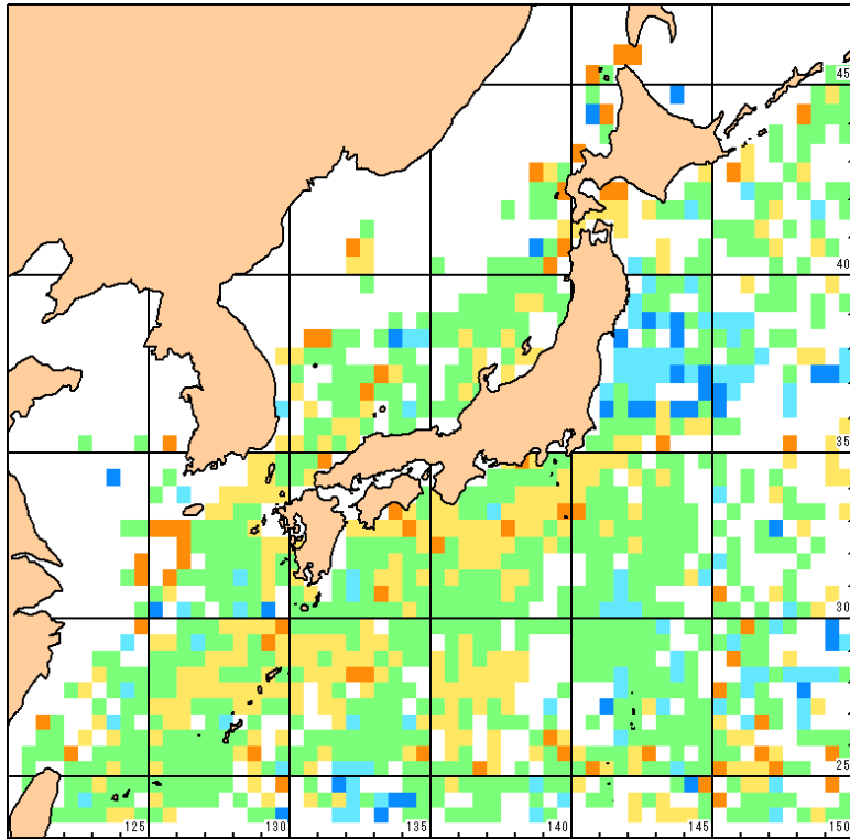
2004年1月水温平年差
