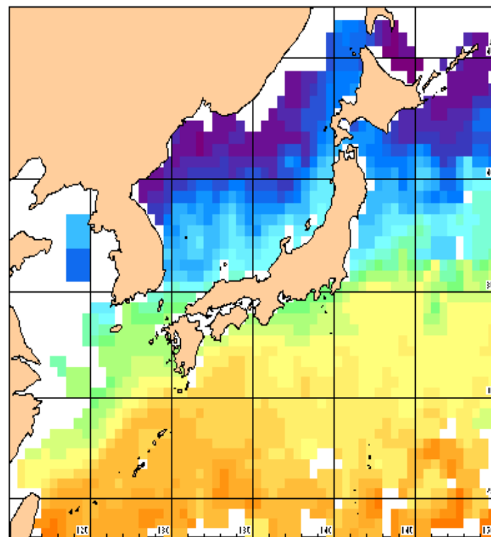
1月の水温平年値( ) 日本海洋データセンターの統計値
