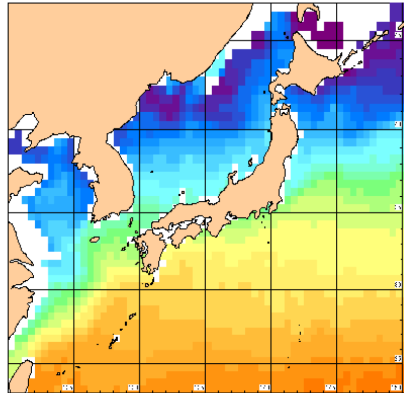
1月の水温平年値( )
