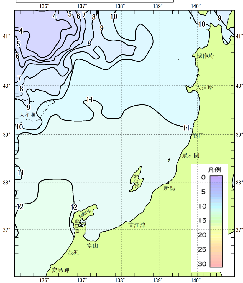
水温水平分布図 表面水温(°C)
