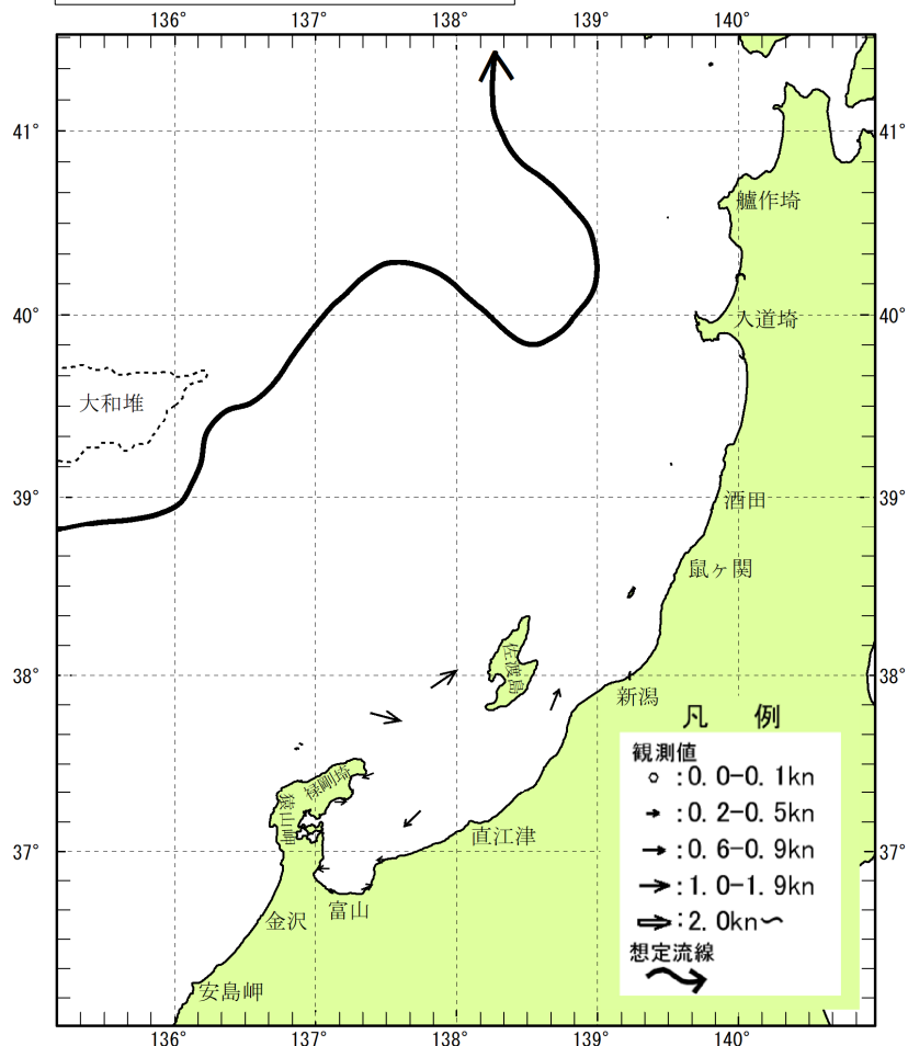
海流図 対馬暖流の流路
