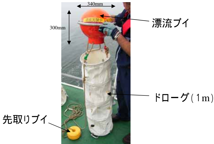
図2 漂流ブイの形状
