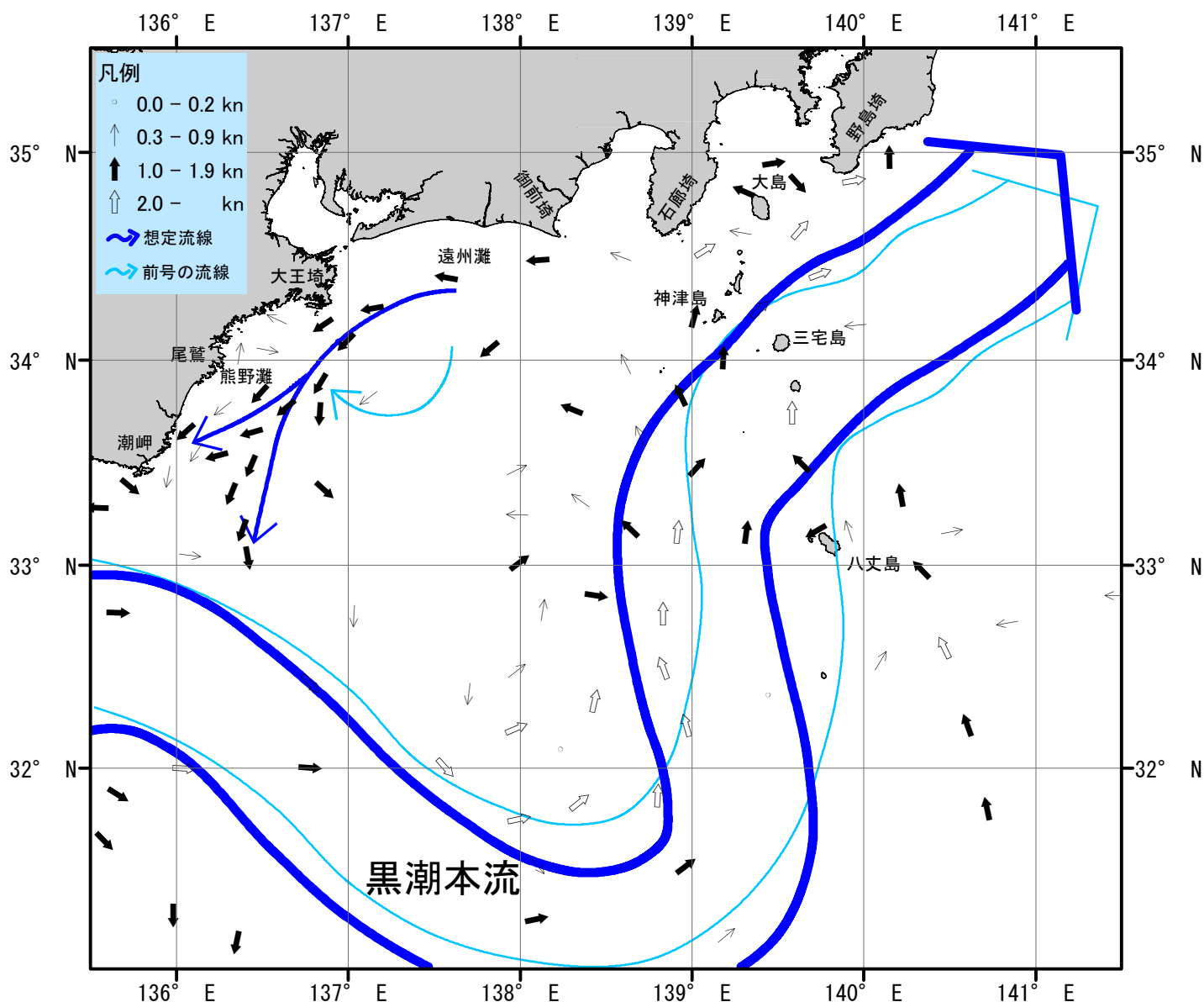
海流図（観測期間：平成29年9月22日-平成29年10月12日）
