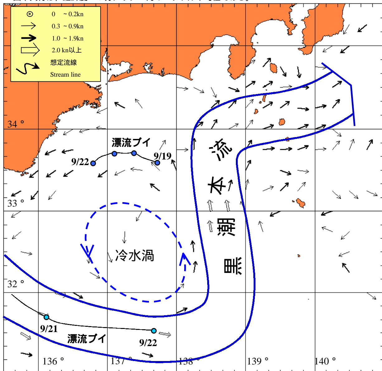
海流図 (観測期間 : 平成16年9月13日~平成16年9月22日)
