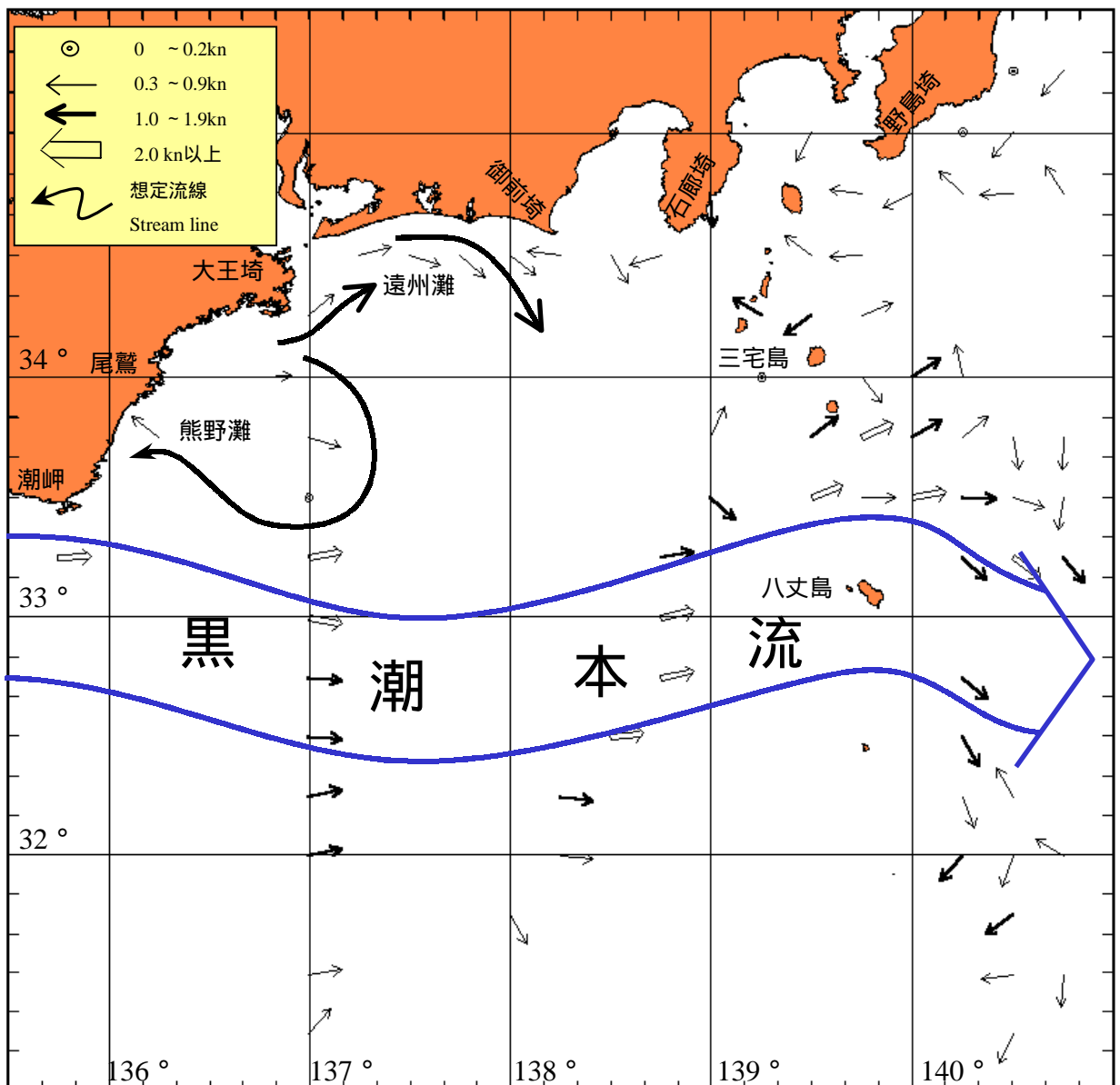
海流図(観測期間：平成13年12月4日～12月13日)
