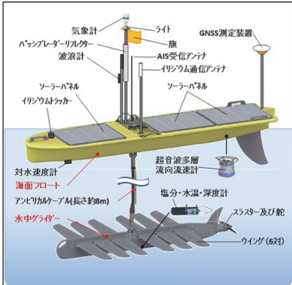
図1 自律型海洋観測装置 (AOV) 長さ約3m
