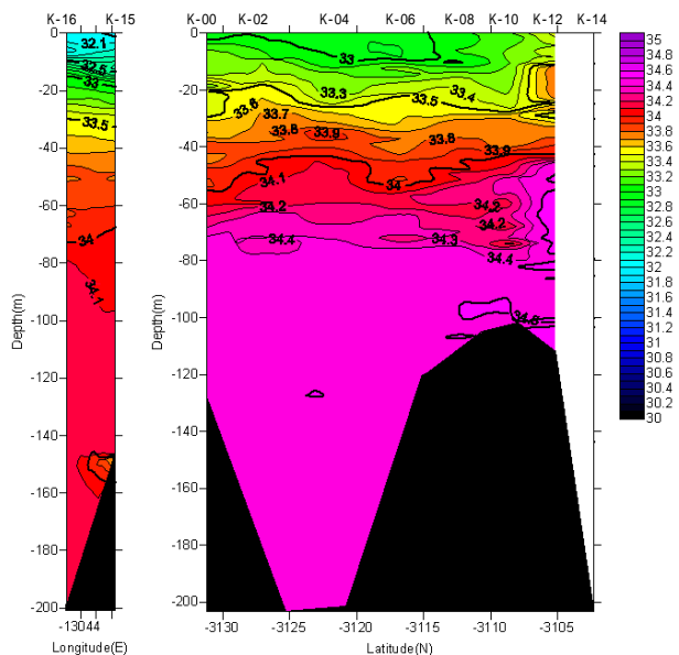
塩分鉛直断面図(2005/07/28-07/29)
