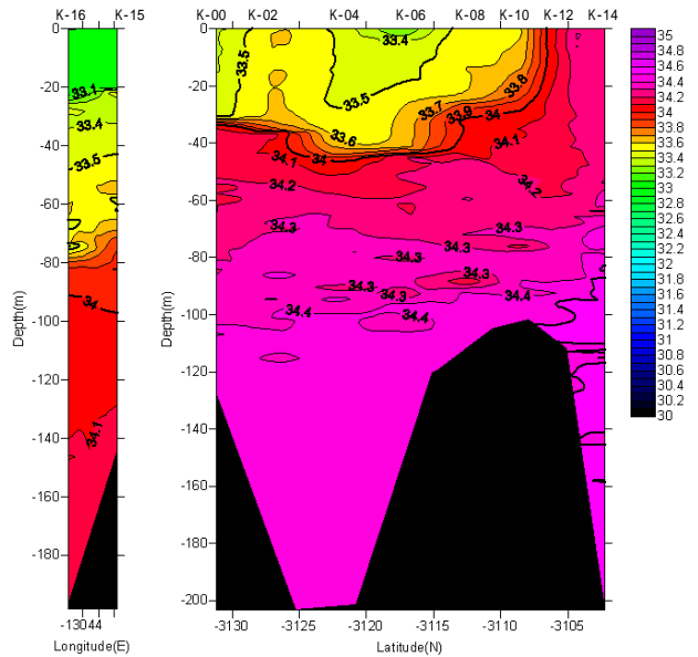
塩分鉛直断面図 (2005/11/15-11/16)
