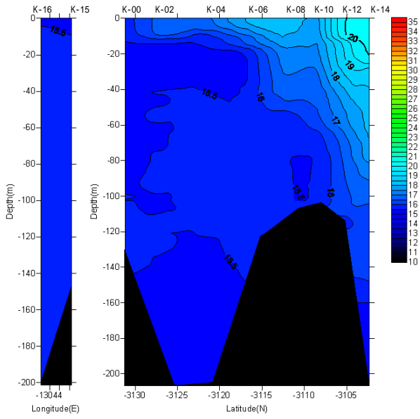
水温鉛直断面(2006/02/23-02/24)
