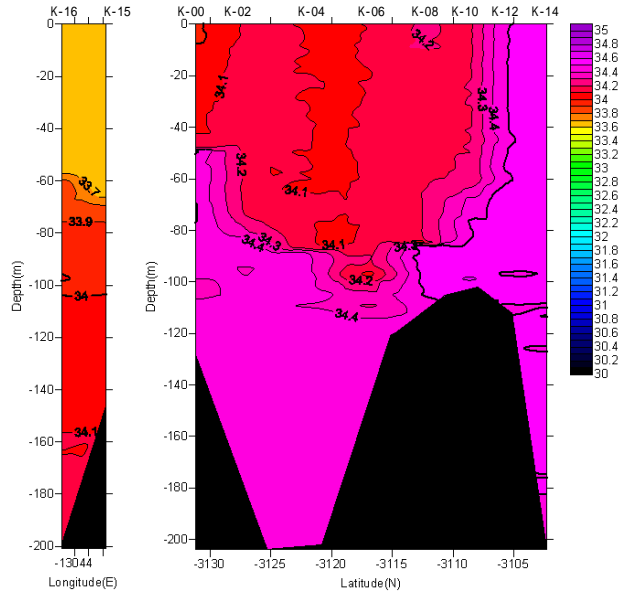
塩分鉛直断面図 (2005/12/19-12/20)
