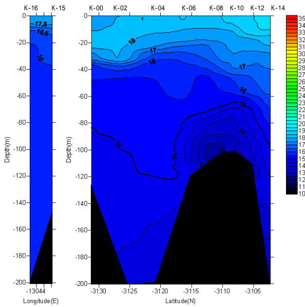
水温鉛直断面(2005/04/19-04/20)
