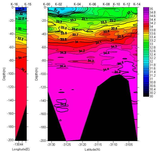
塩分鉛直断面図(2005/08/29-08/30)
