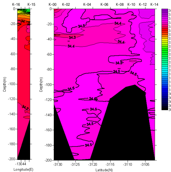
塩分鉛直断面図(2005/04/19-04/20)
