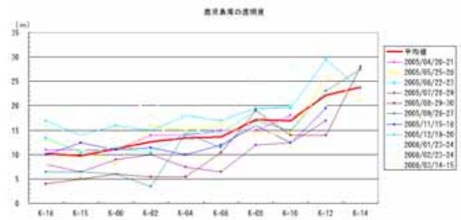
7図 鹿児島湾の透明度
