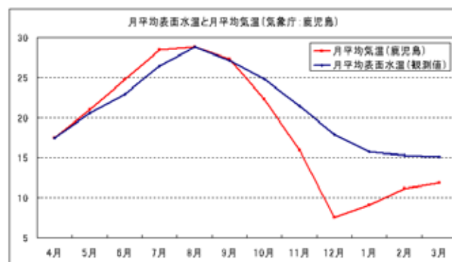
3図 月平均水温と月平均気温
