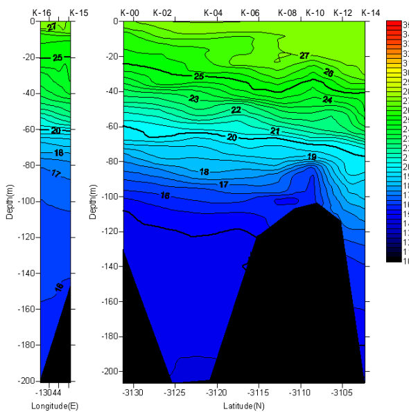
水温鉛直断面(2005/09/26-09/27)
