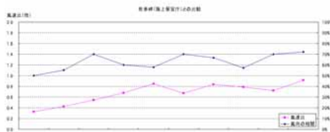
6図 佐多岬との風データの比較
