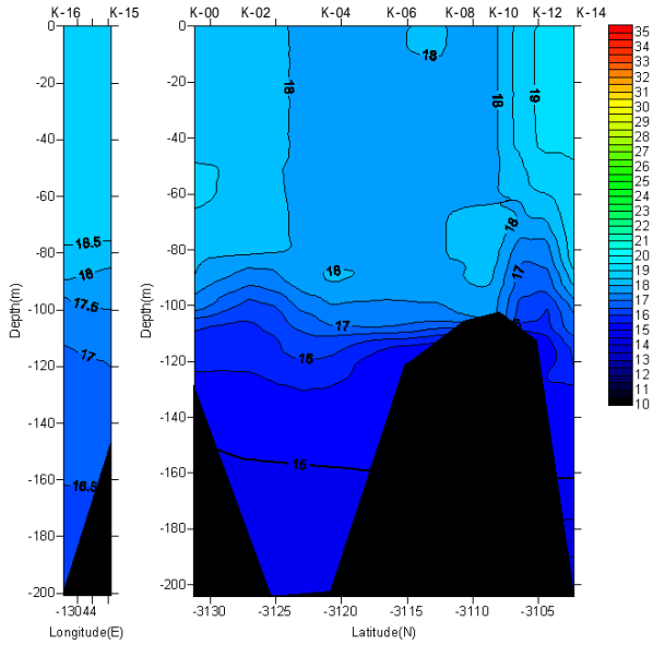
水温鉛直断面 (2005/12/19-12/20)
