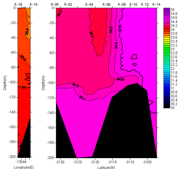
塩分鉛直断面図 (2006/01/23-01/24)
