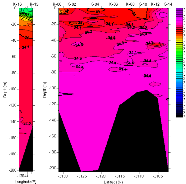
塩分鉛直断面図(2005/05/25-05/26)
