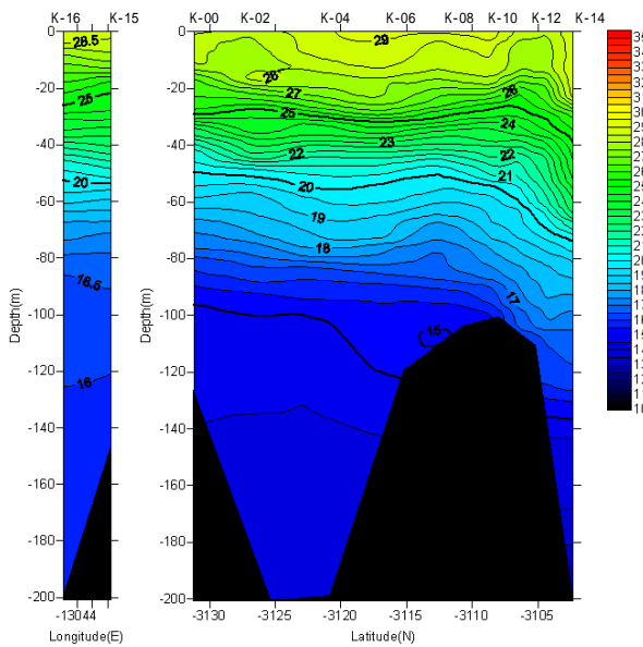
水温鉛直断面(2005/08/29-08/30)
