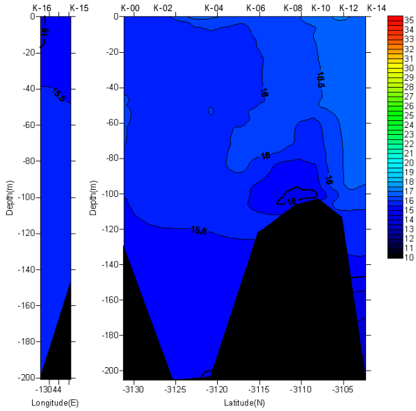
水温鉛直断面(2006/03/14-03/15, 03/24)
