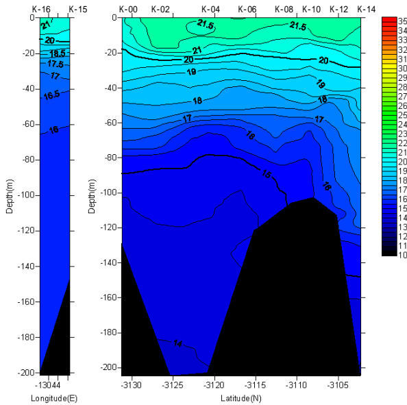
水温鉛直断面(2005/05/25-05/26)
