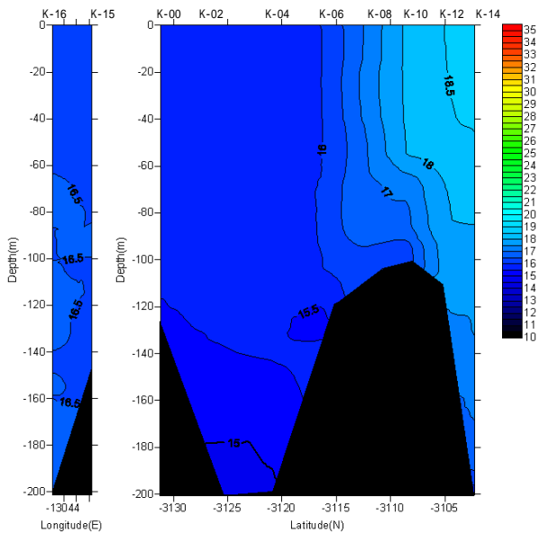
水温鉛直断面 (2006/01/23-01/24)
