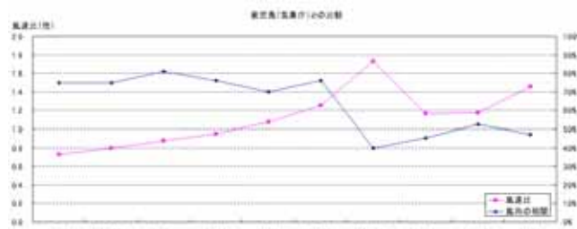
5図 鹿児島との風データの比較
