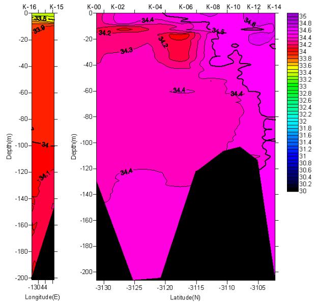
塩分鉛直断面図(2006/02/23-02/24)
