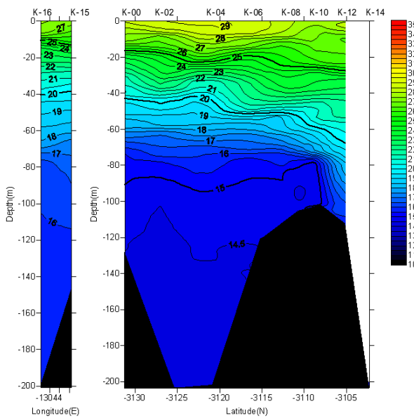
水温鉛直断面(2005/07/28-07/29)
