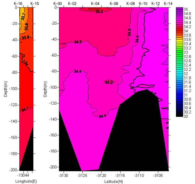
塩分鉛直断面図(2006/03/14-03/15, 03/24)
