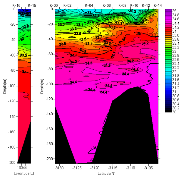
塩分鉛直断面図(2005/09/26-09/27)
