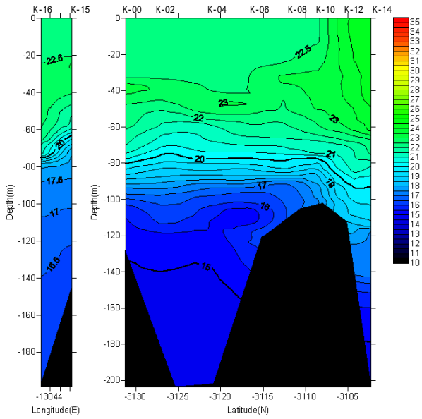
水温鉛直断面 (2005/11/15-11/16)
