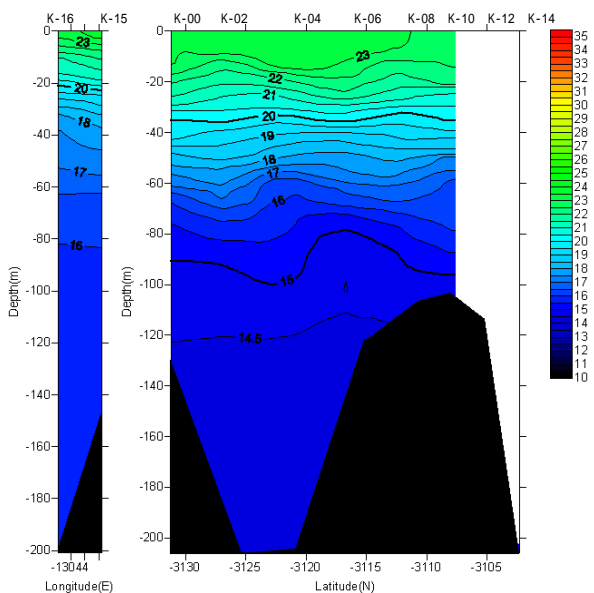
水温鉛直断面(2005/06/22-06/23)
