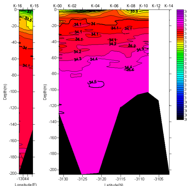
塩分鉛直断面図(2005/06/22-06/23)
