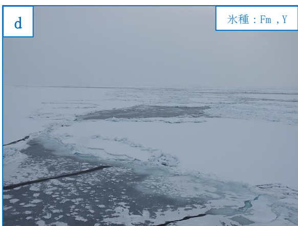
図8.10 令和4年2月14日の海水写真
