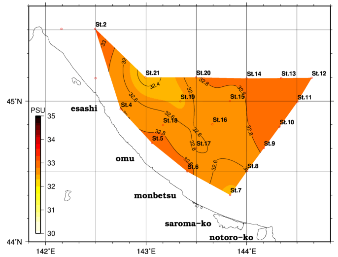
図3.3 水温及び塩分水平分布図（水深50m層）
