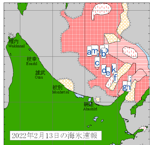
図8.9 令和4年2月13日の海氷写真
