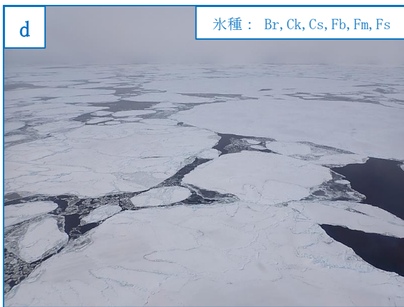
図8.7 令和4年2月13日の海氷写真
