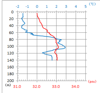
図2 各観測点の水温及び塩分鉛直分布図 [1/2]
