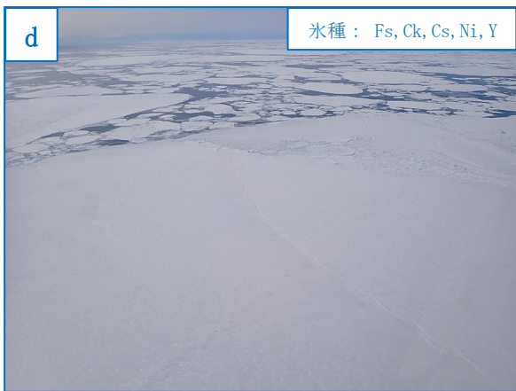
図8.12 令和4年2月15日の海氷写真
