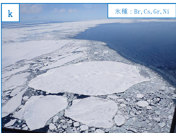
図8.13 令和4年2月15日の海氷写真
