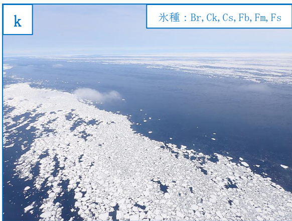
図8.8 令和4年2月13日の海氷写真
