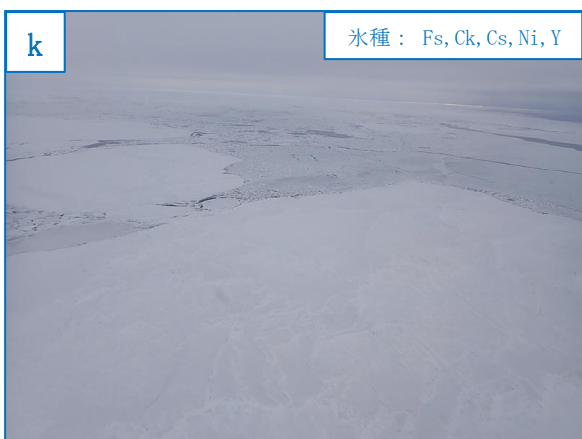
図8.2 令和4年2月11日の海氷写真
