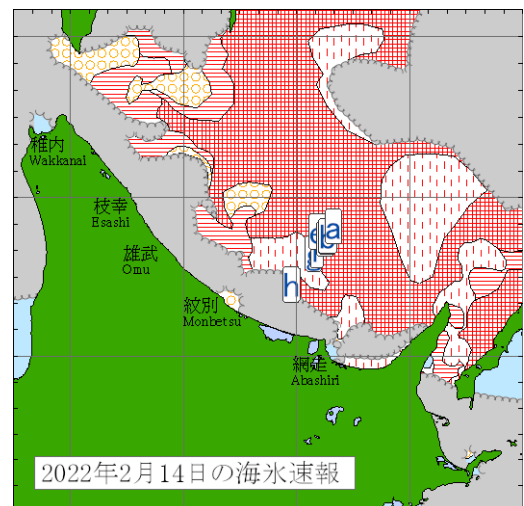
図8.11 令和4年2月14日の海氷写真
