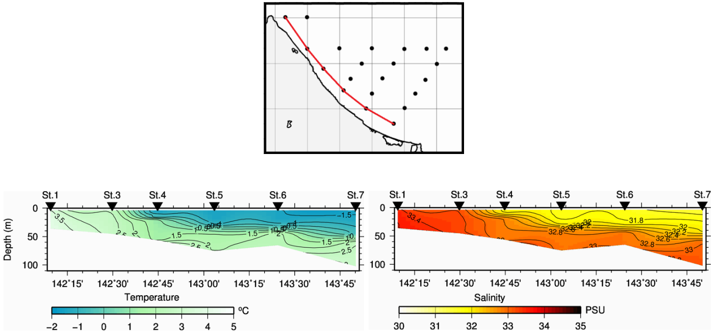
図4.4 水温及び塩分鉛直断面図 (L1線)
