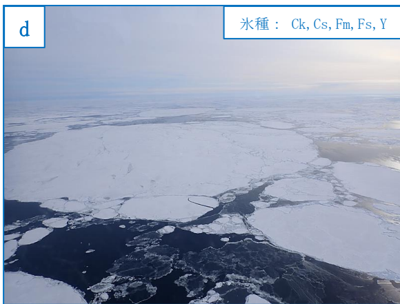
図8.4 令和4年2月12日の海氷写真
