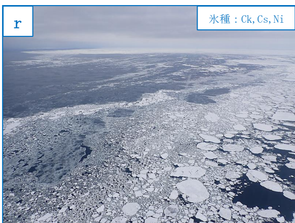
図8.3 令和4年2月11日の海氷写真
