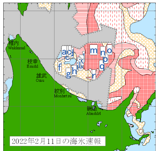
図8.2 令和4年2月11日の海氷写真
