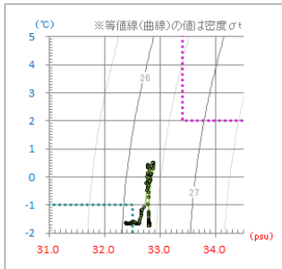
図5 各観測点のT-S図 [1/2]
